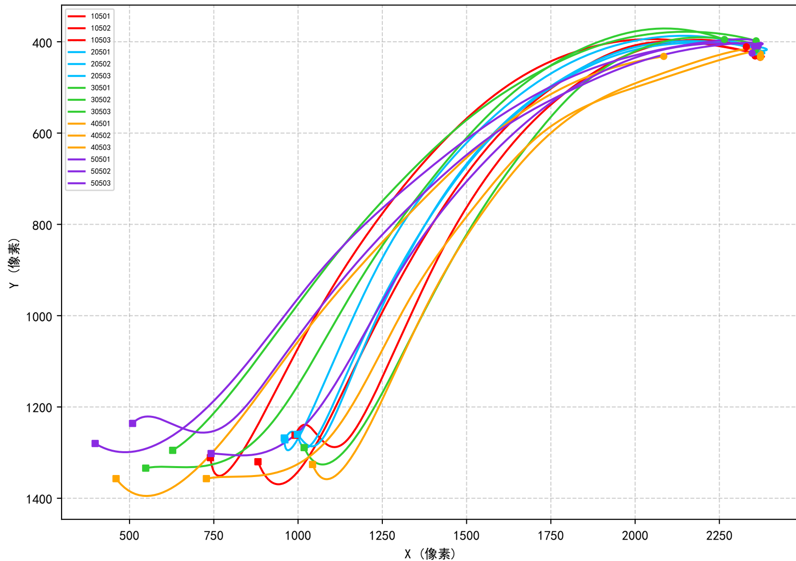
实验组 b=5 所有飞行轨迹 (同a同色)
