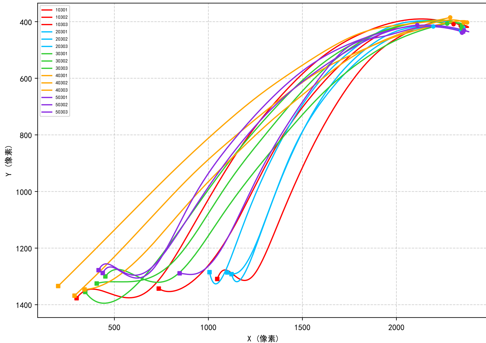
实验组 b=3 所有飞行轨迹 (同a同色)
