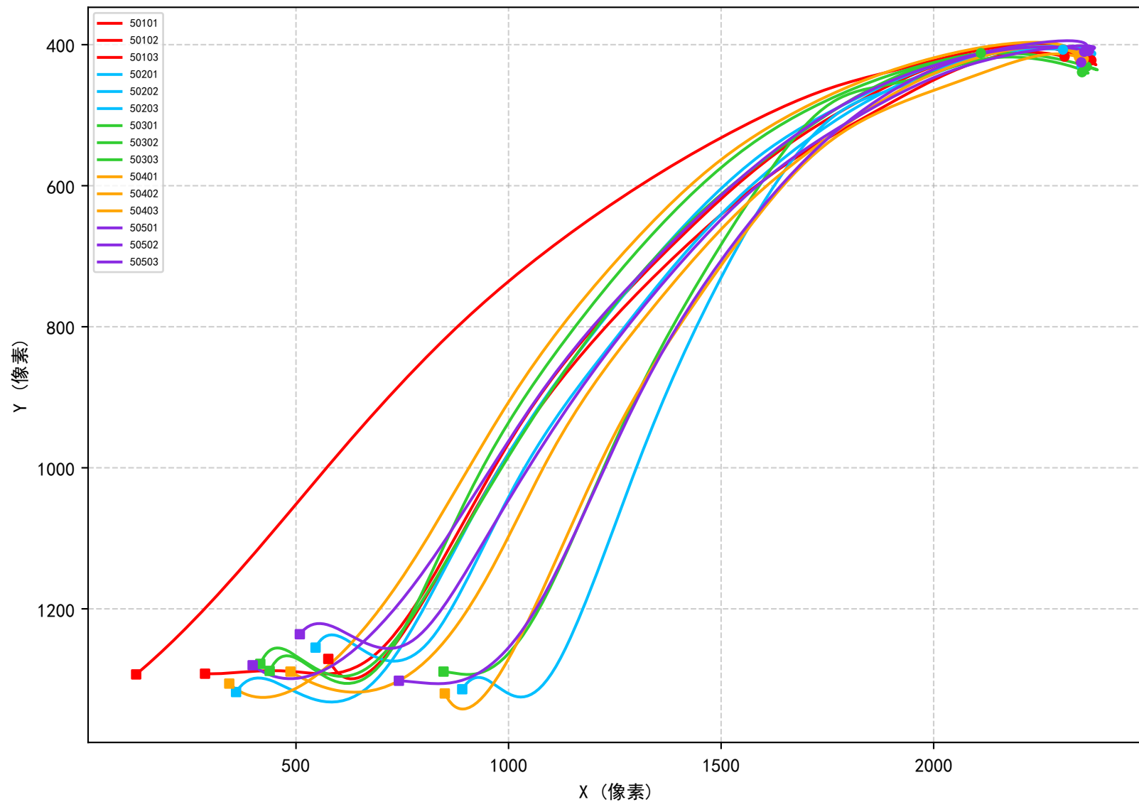
实验组 a=5 所有飞行轨迹 (同b同色)
