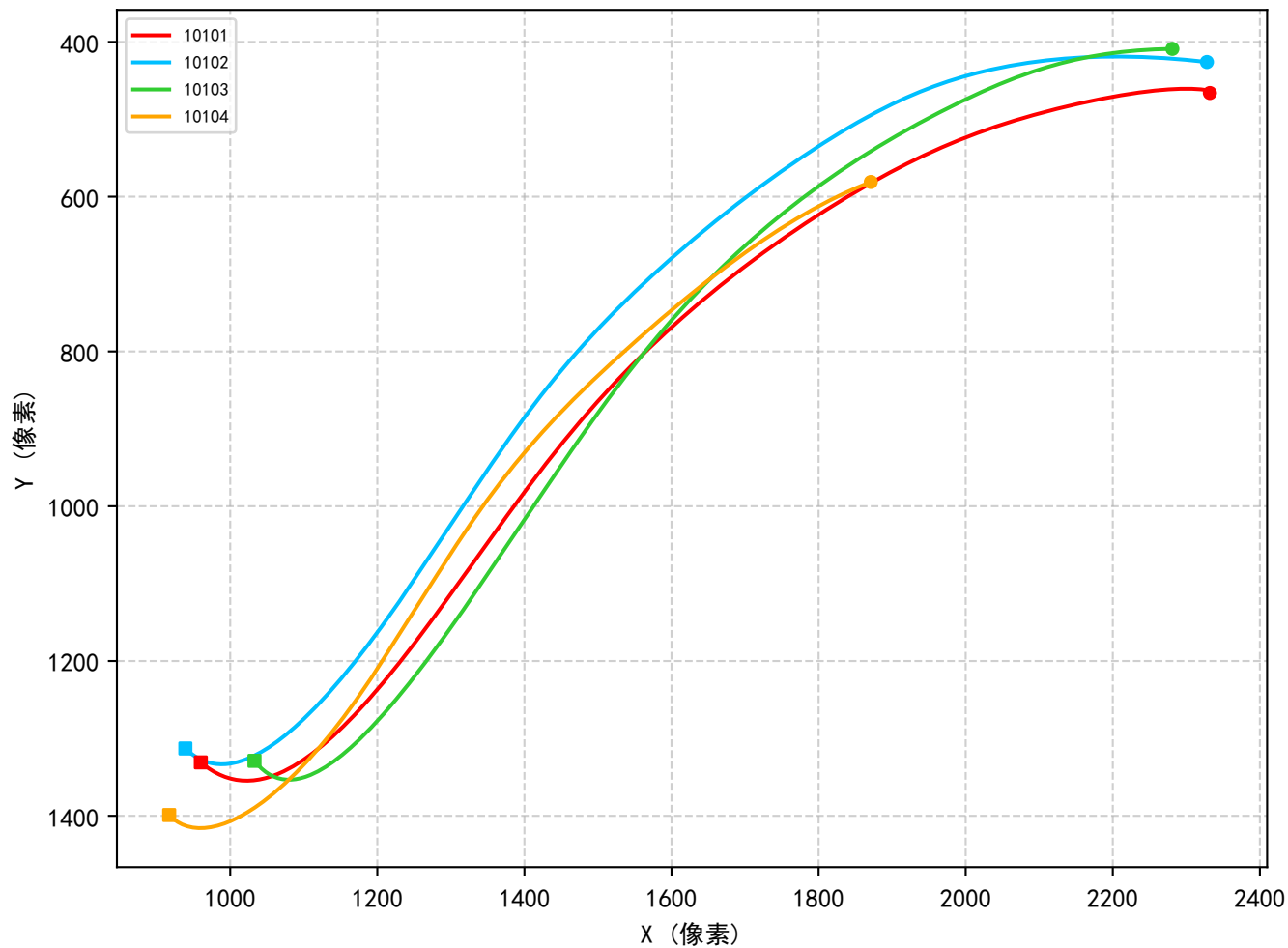
实验组 101 各次飞行对比
