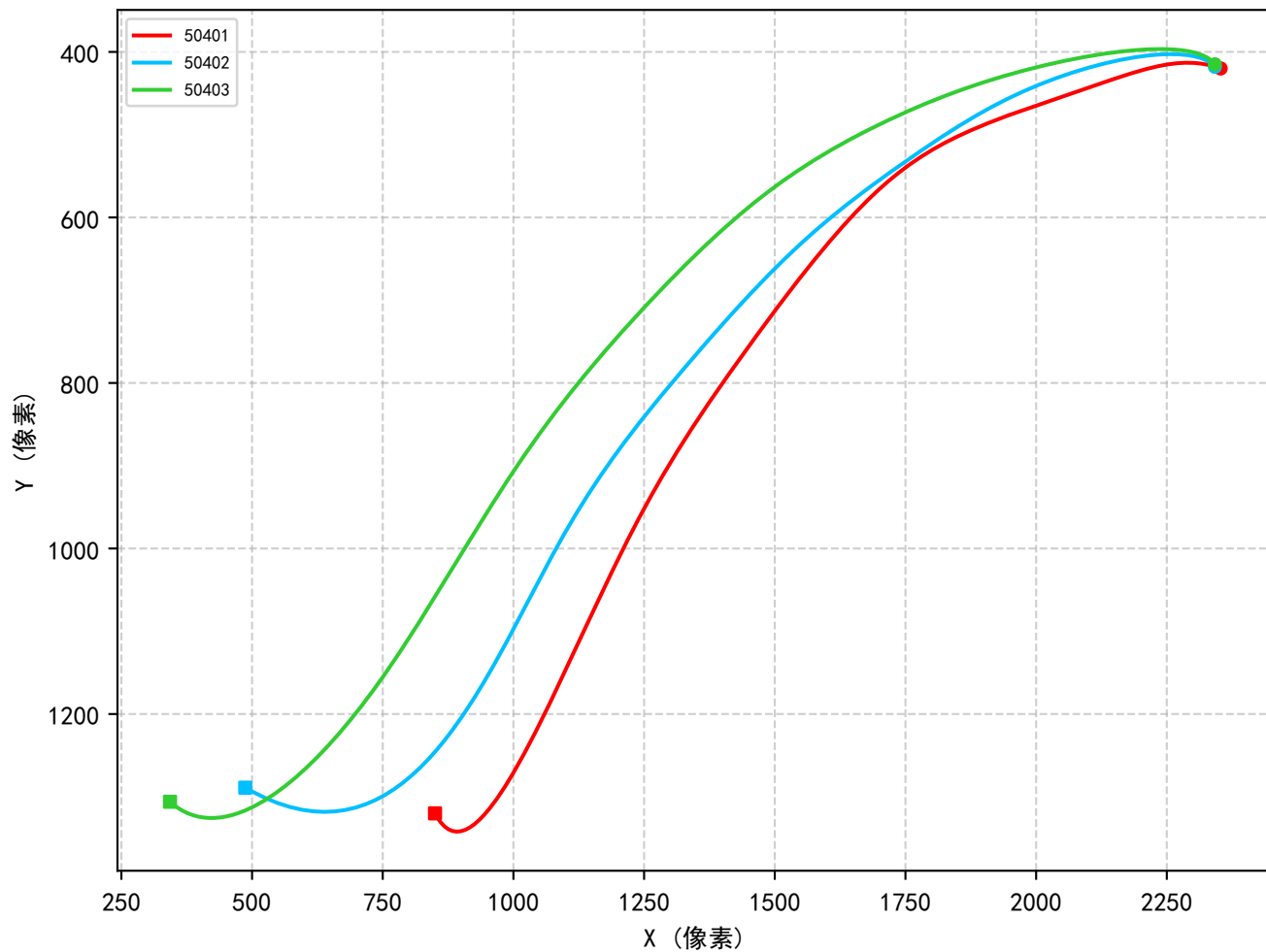
实验组 504 各次飞行对比
