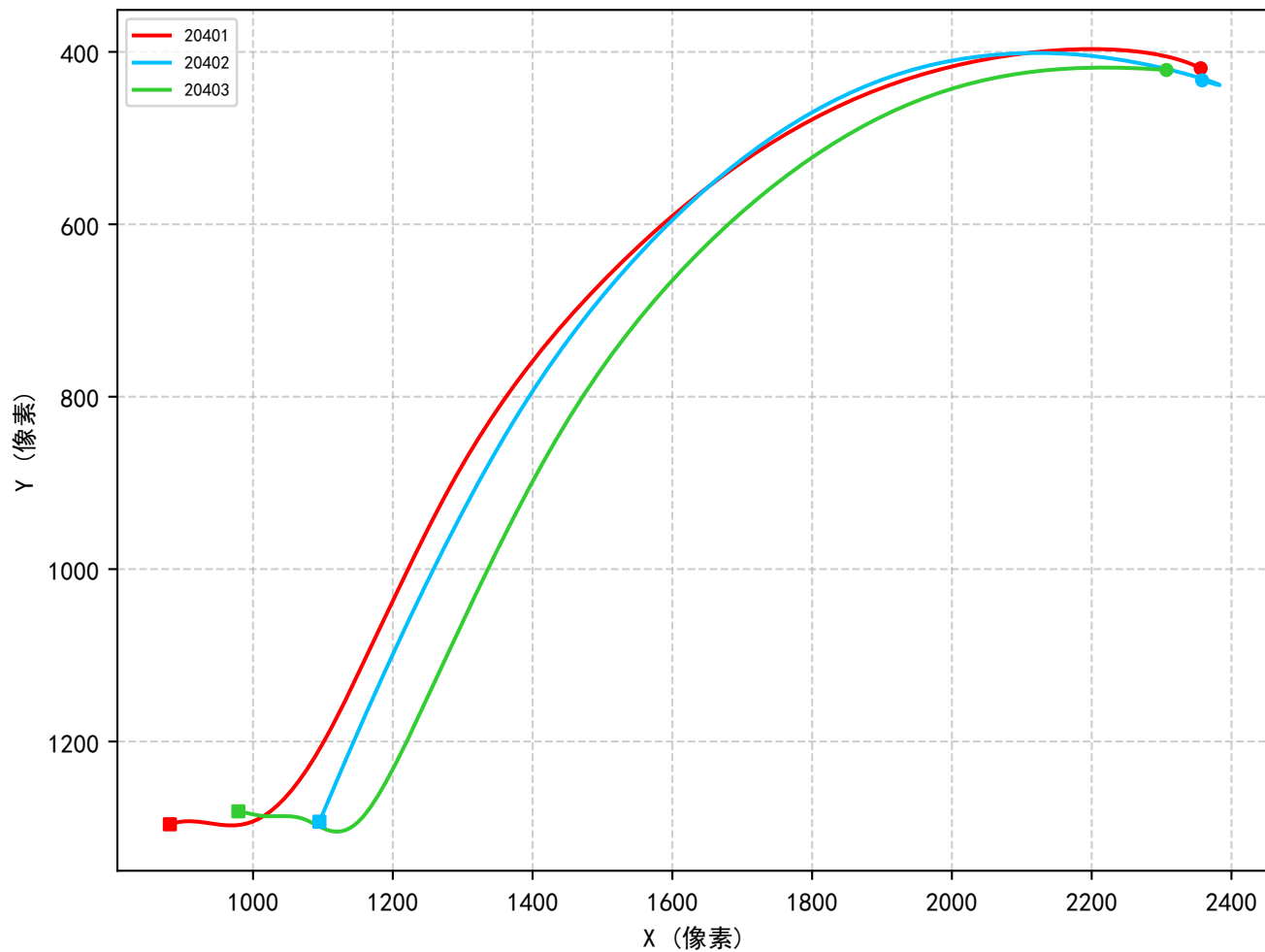
实验组 204 各次飞行对比
