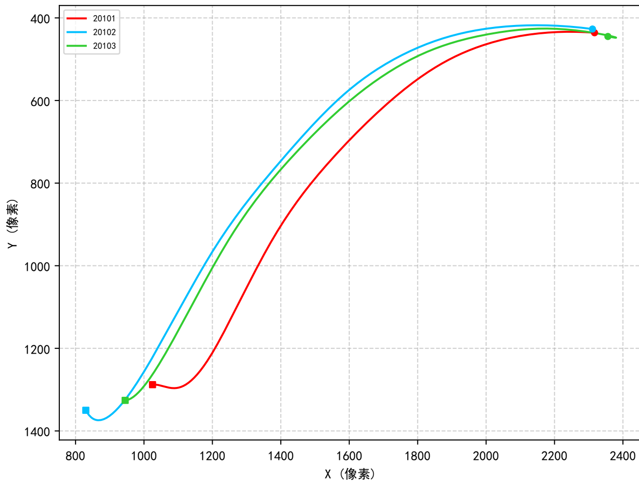
实验组 201 各次飞行对比
