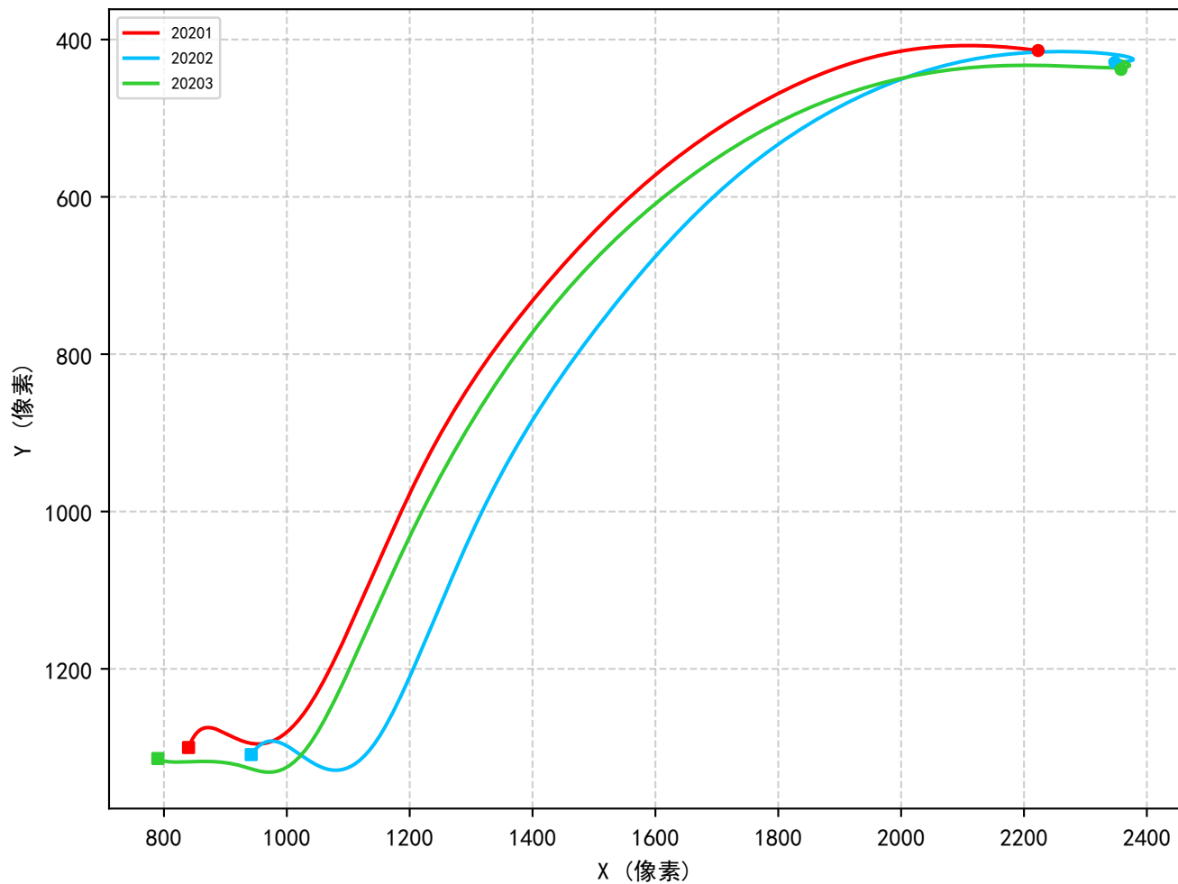
实验组 202 各次飞行对比
