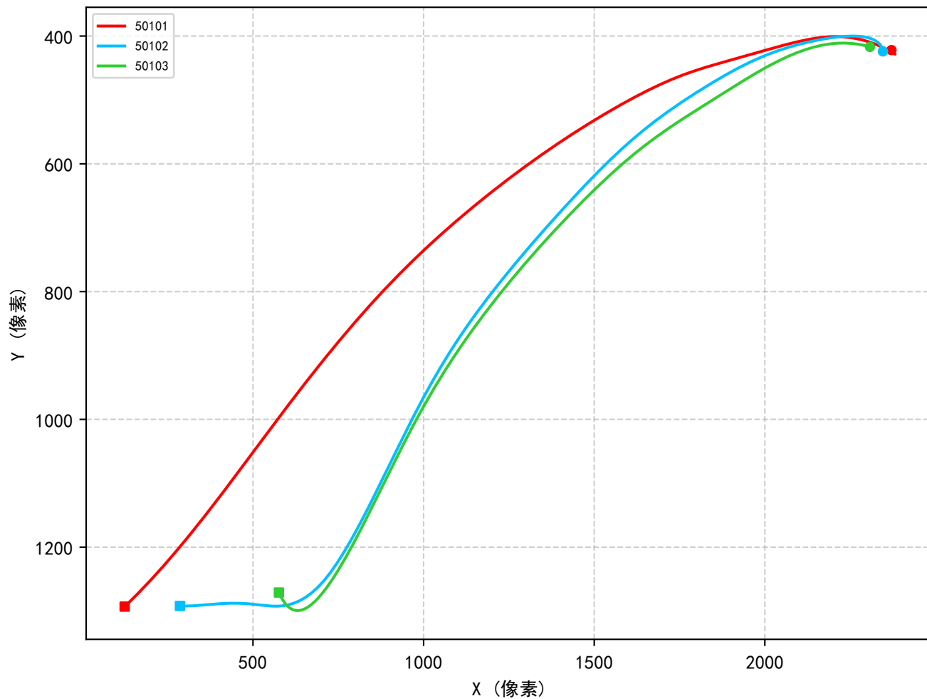
实验组 501 各次飞行对比
