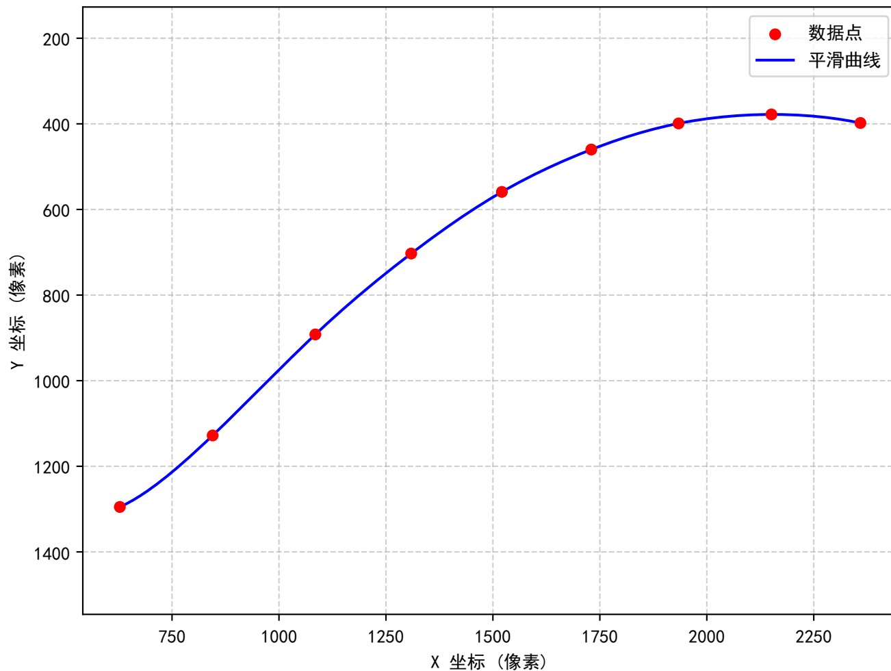
实验 30503 纸飞机轨迹
