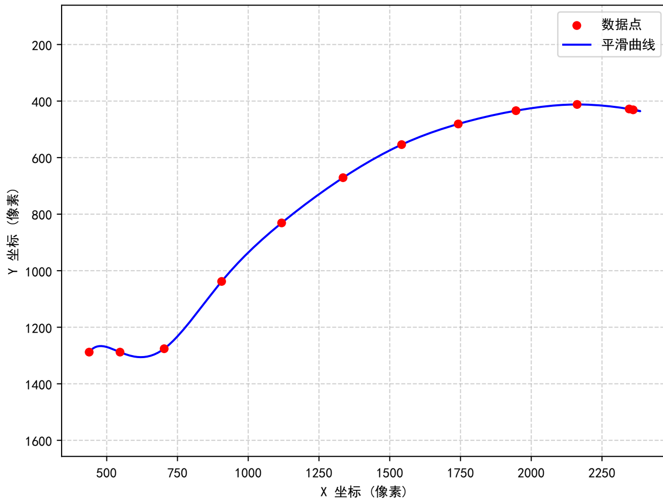
实验 50302 纸飞机轨迹
