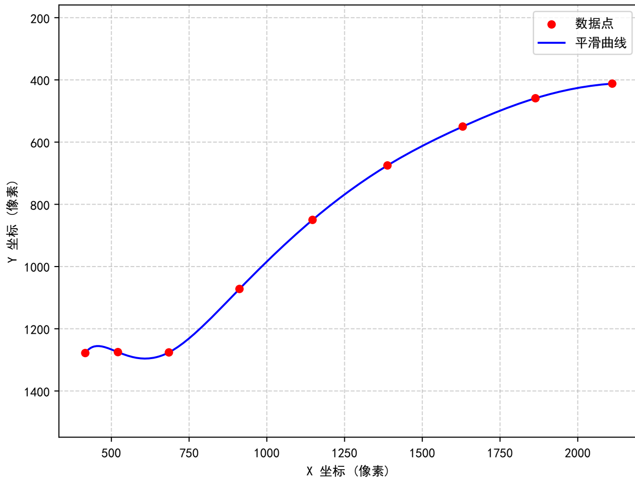
实验 50301 纸飞机轨迹
