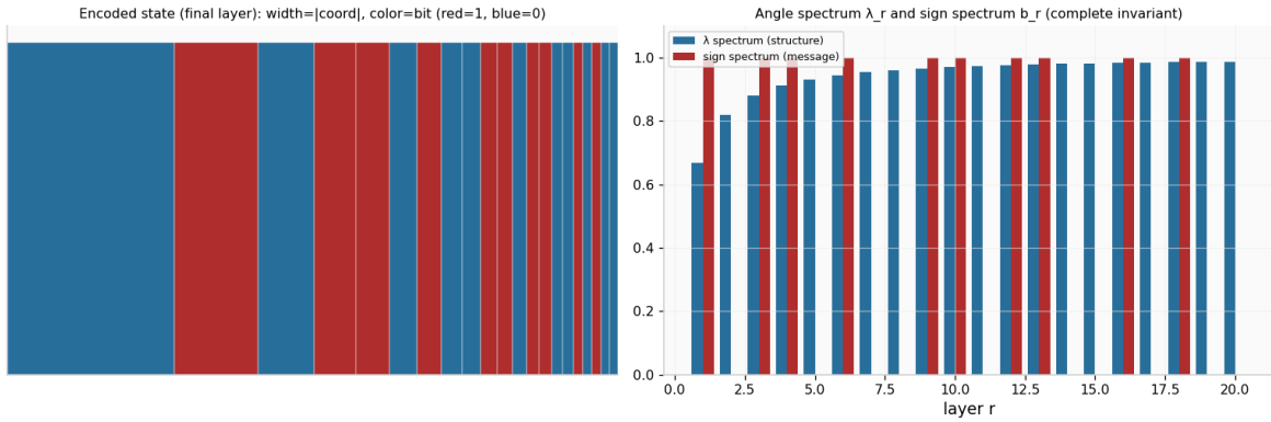
图1 编码后结构。左：20 比特消息的最终状态——块宽 = |P_k| （上下文包络），颜色 = 符号谱（红 = 1，蓝 = 0）；注意左端最早比特的块宽显著大于右端（定理 6.2 的对数剖面）。右：角度谱 \lambda_r （结构，单调趋 1）与符号谱 b_r （消息）——由定理 7.2，两者构成状态的完备描述。
