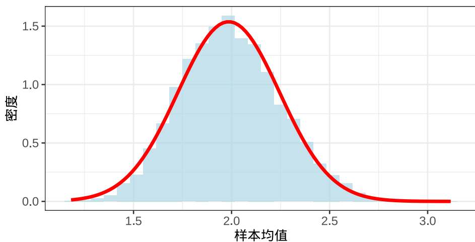
中心极限定理: 伽马分布
