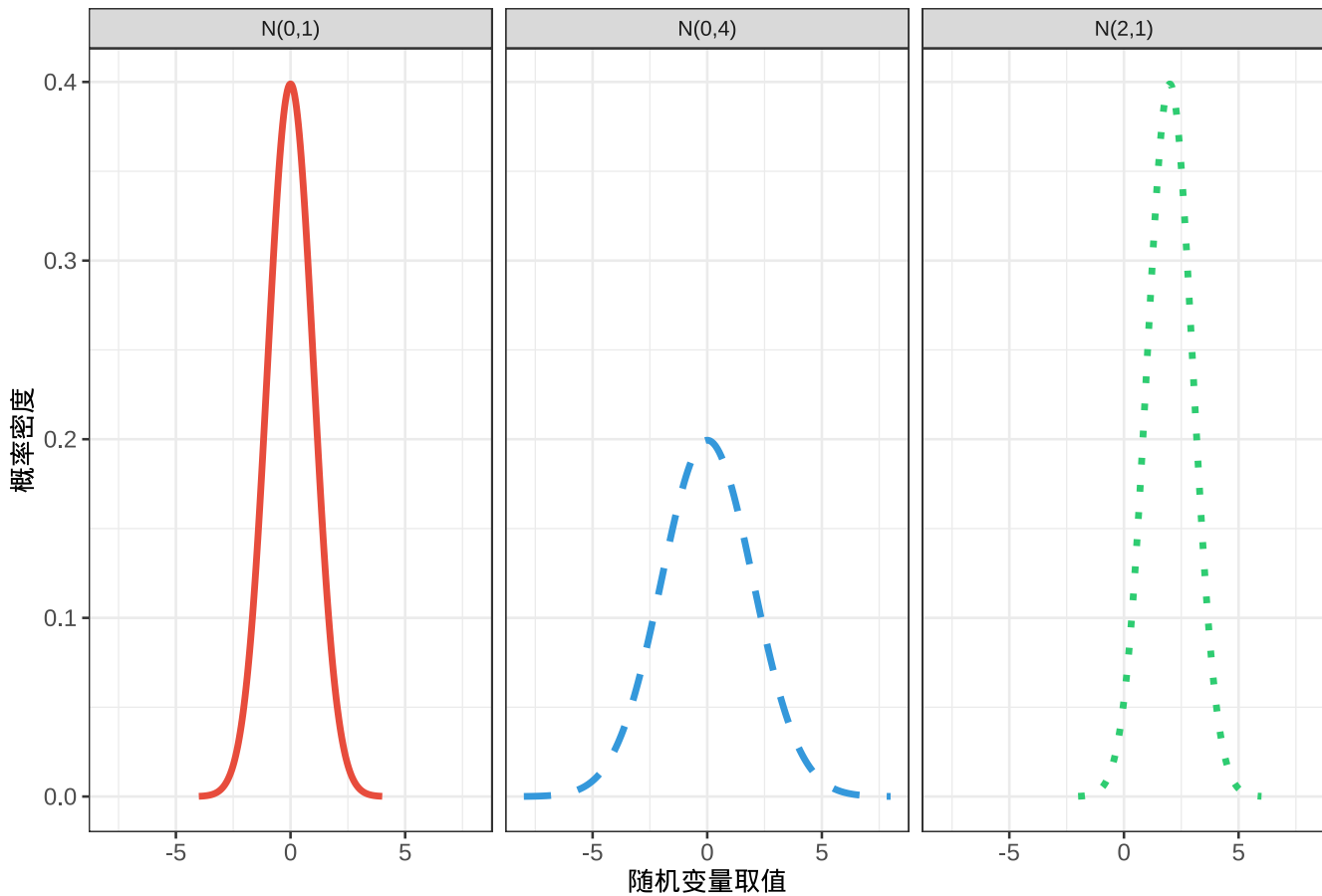
正态分布：不同参数组合的概率密度函数
