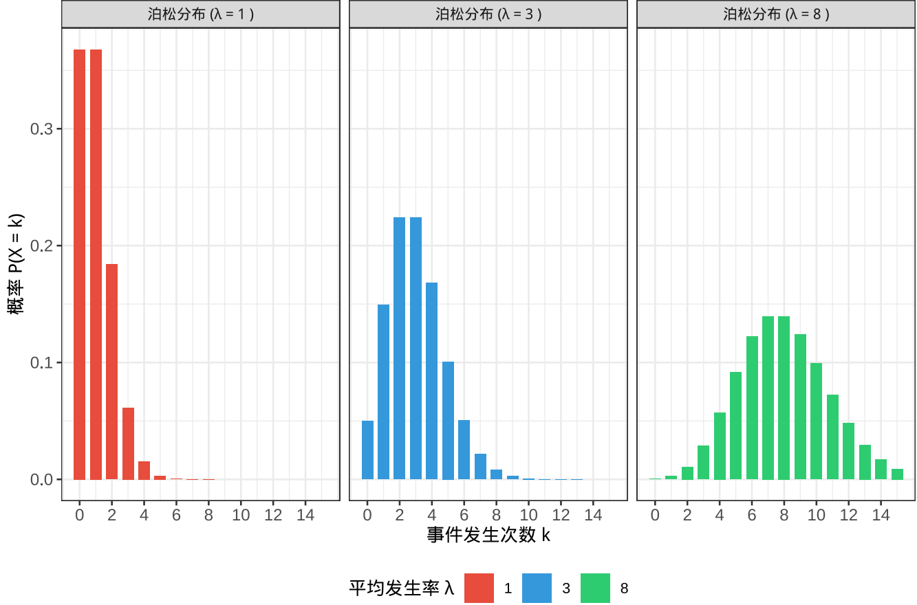
泊松分布：不同平均发生率下的概率分布
