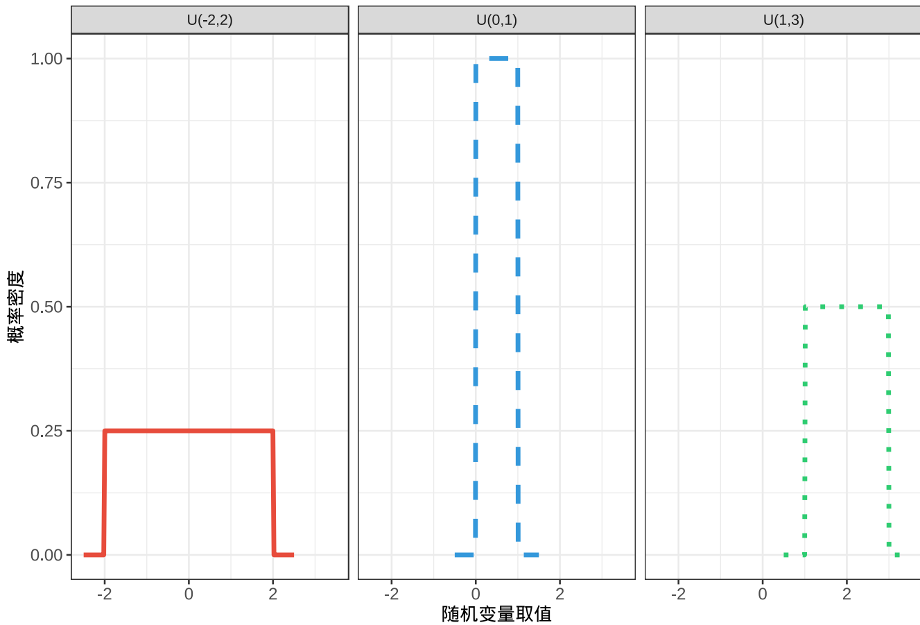
均匀分布：不同区间参数的概率密度函数
