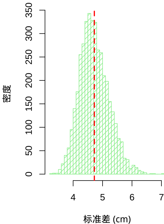
标准差的后验分布
