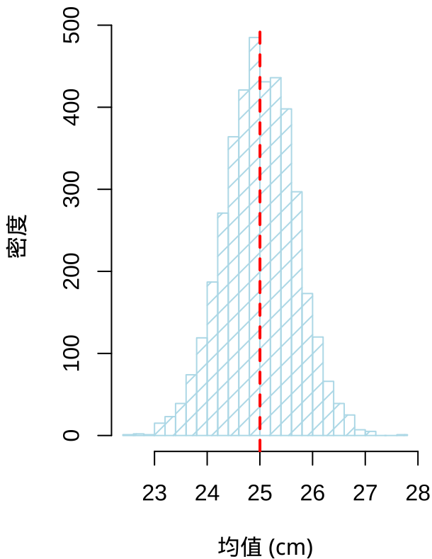
均值的后验分布
