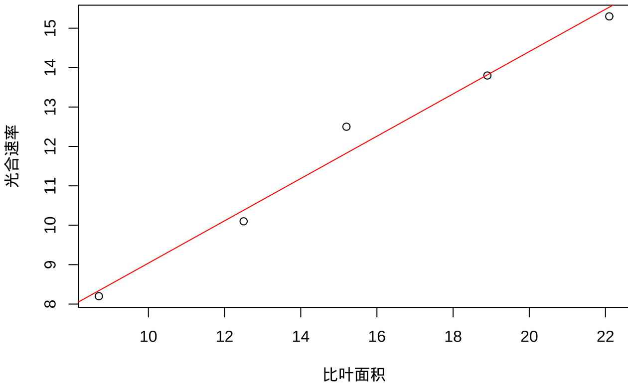
叶片经济型谱：比叶面积与光合速率关系
