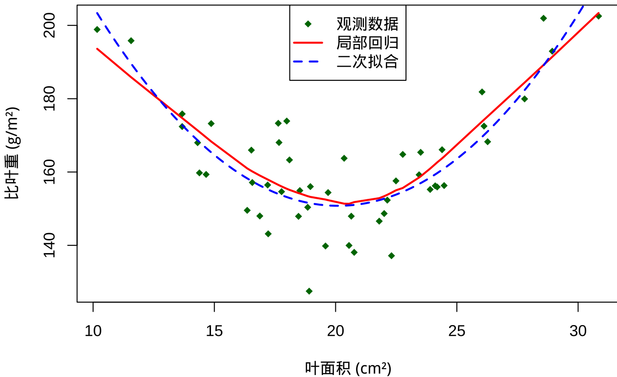
植物功能性状间的非线性关系
