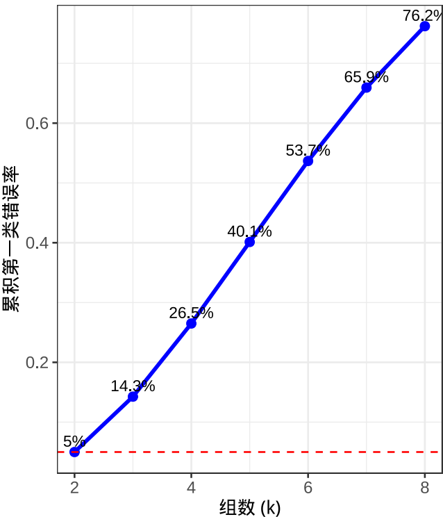
累积第一类错误率
