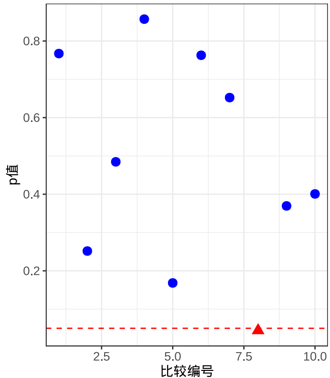
多个t检验：p值分布
