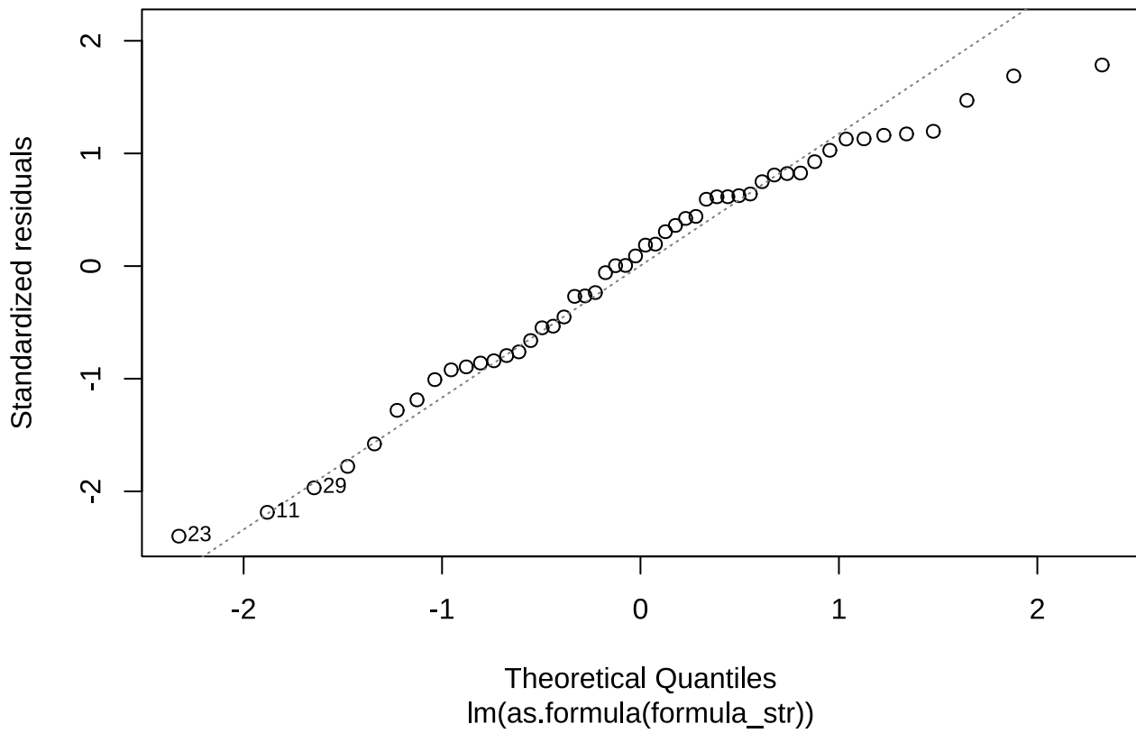
正态Q-Q图 Q-Q Residuals
