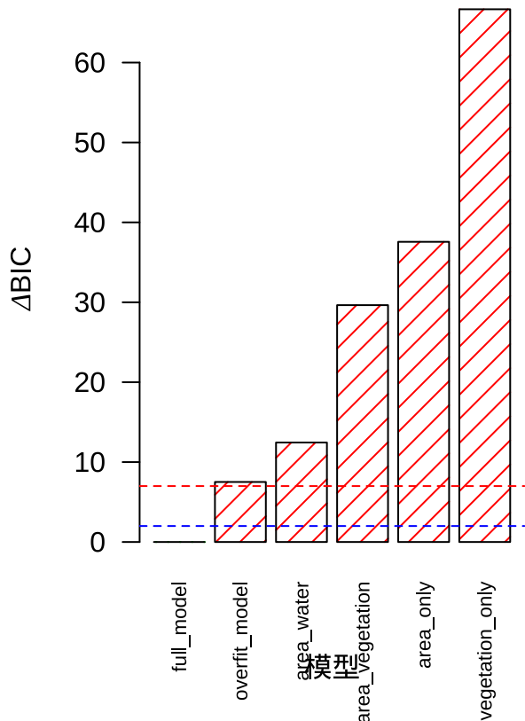
常林的鸟类模型 \Delta BIC 差异比较
