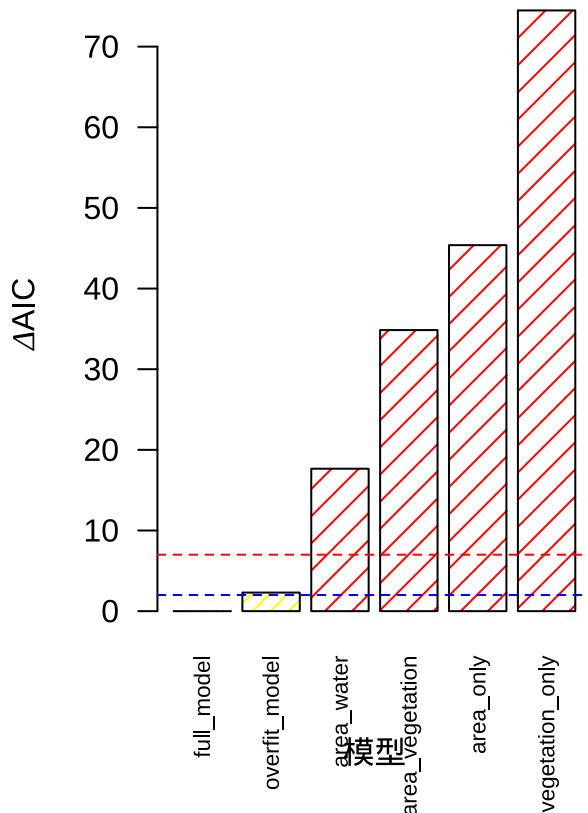
常林的鸟类模型 \Delta AIC 差异比较
