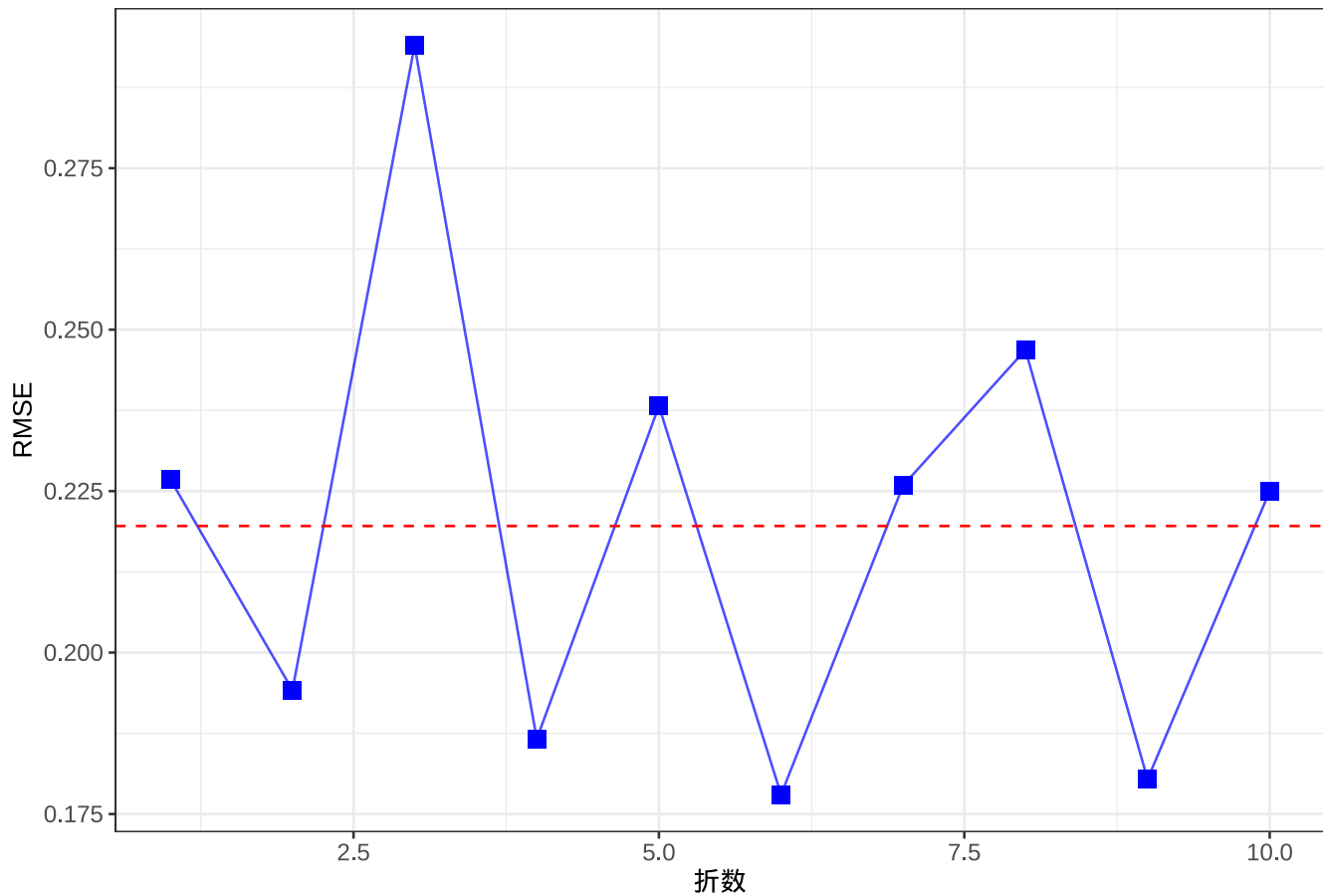
常林的森林鸟类模型10折交叉验证：RMSE变化
