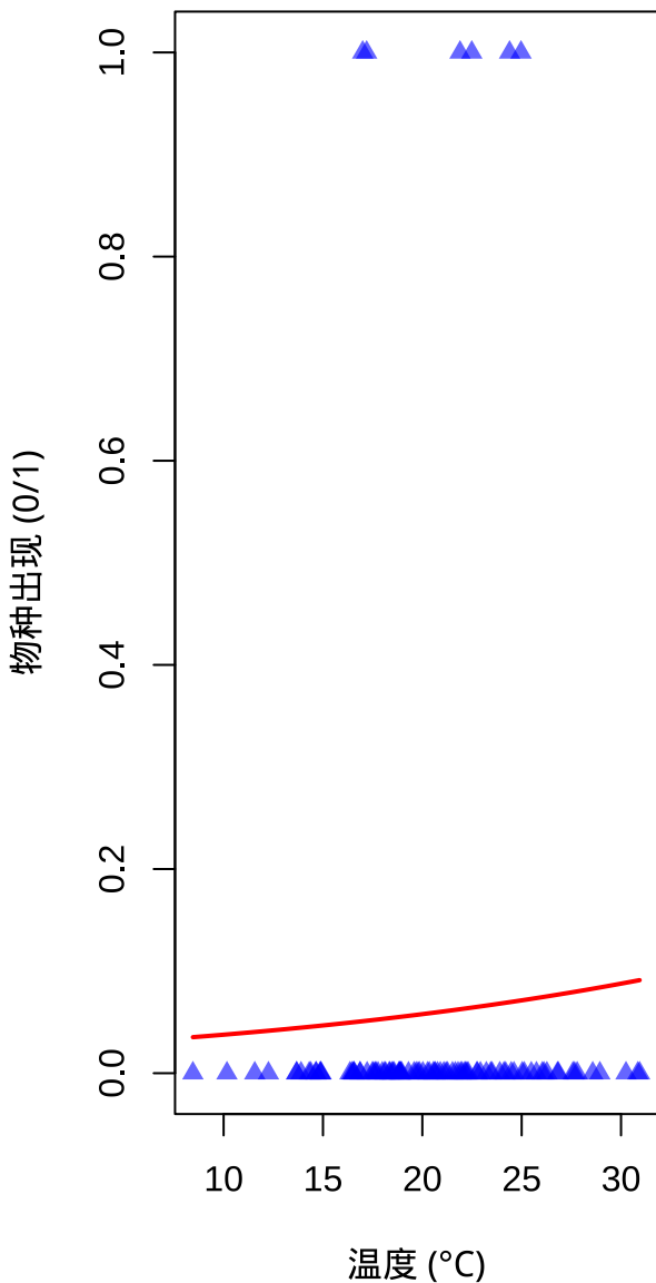
温度与物种出现的关系
