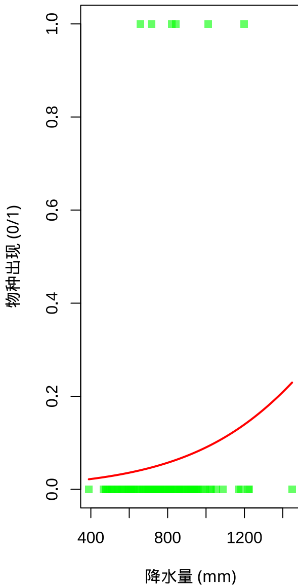
降水量与物种出现的关系
