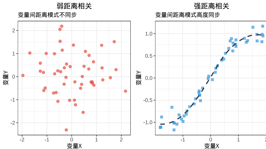
图 4.4 距离相关强弱对比示意图：左图显示弱距离相关，右图显示强距离相关
