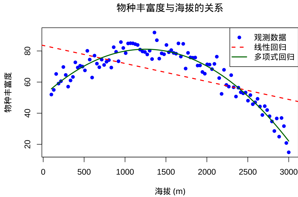
图 7.12 物种丰富度与海拔关系的多项式回归：线性与二次多项式的拟合对比。
