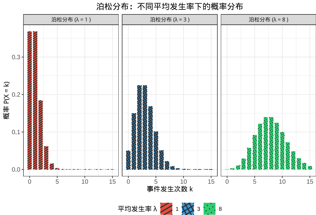
图 2.13 泊松分布：不同平均发生率下稀有事件发生次数的概率分布
