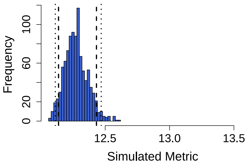
图 6.6 物种共现零模型检验: EcoSimR 包分析结果
