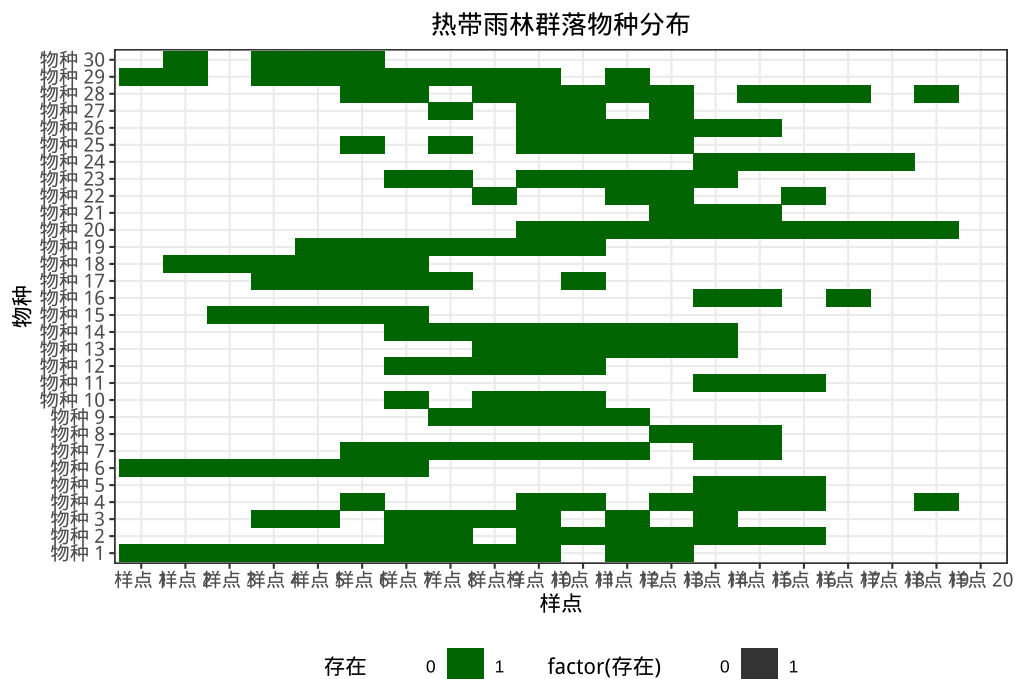
图 6.2 热带雨林群落物种分布 heatmap：基于环境梯度的物种分布模式。使用颜色和透明度组合表示物种存在状态
