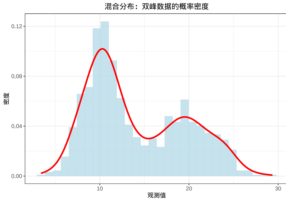
图 2.20 混合分布：双峰数据的概率密度函数
