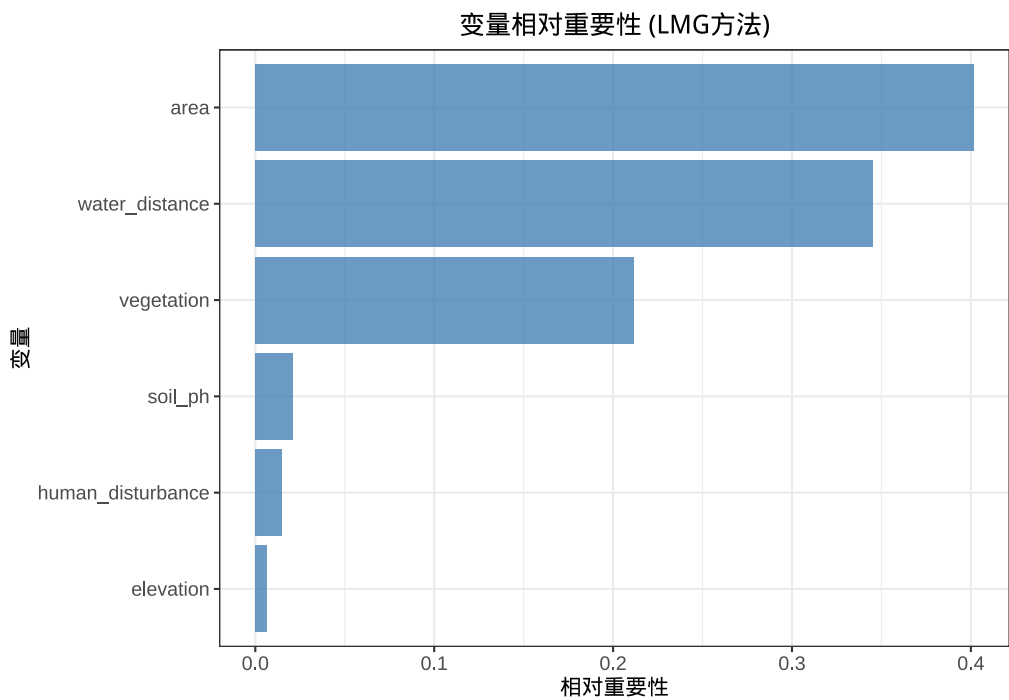
图 7.9 变量相对重要性柱状图：使用 LMG 方法计算的各预测变量对模型解释的相对贡献度
