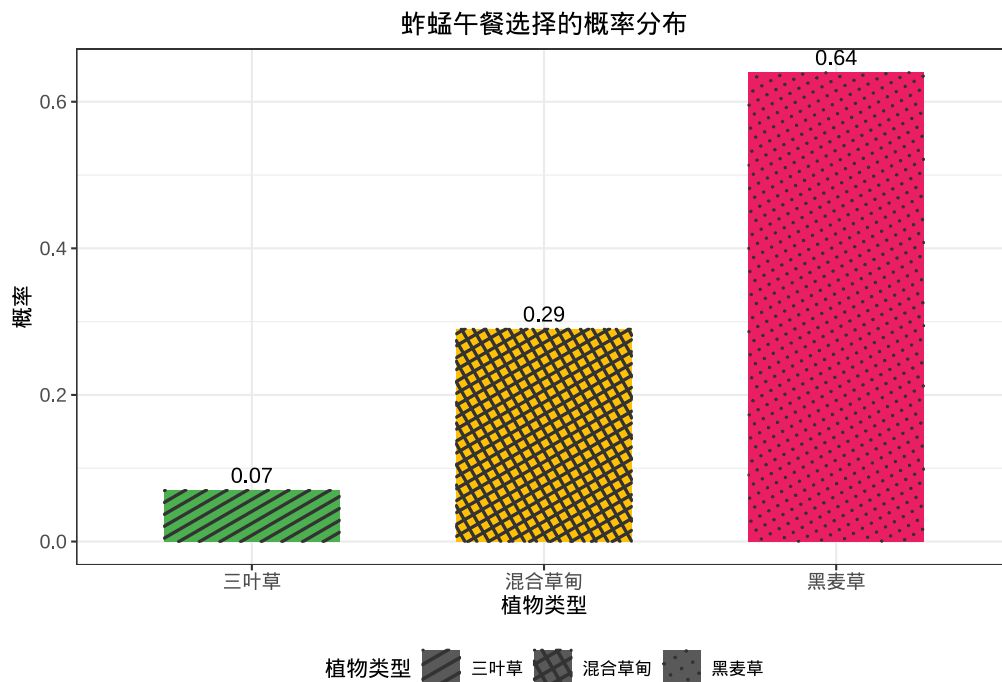
图 2.9 蚱蜢午餐选择的概率分布：三种草地的选择概率对比。
