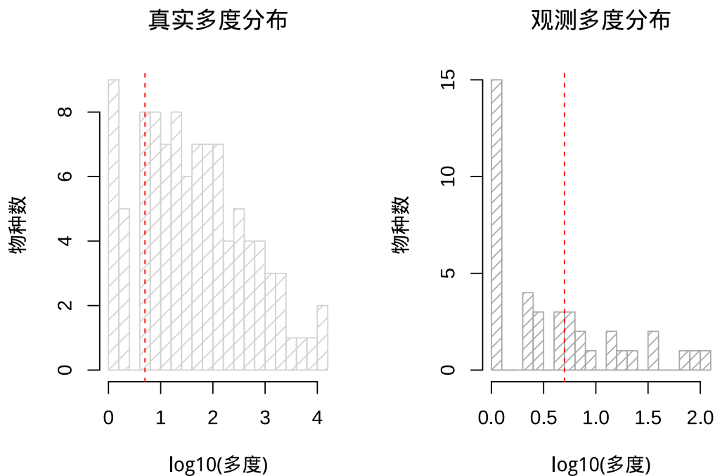
图 3.13 稀有种对多样性估计的影响：真实群落（左）与观测群落（右）的分布对比。
