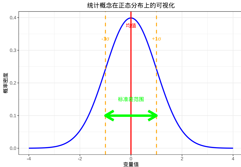
图 2.23 统计概念在正态分布上的可视化
