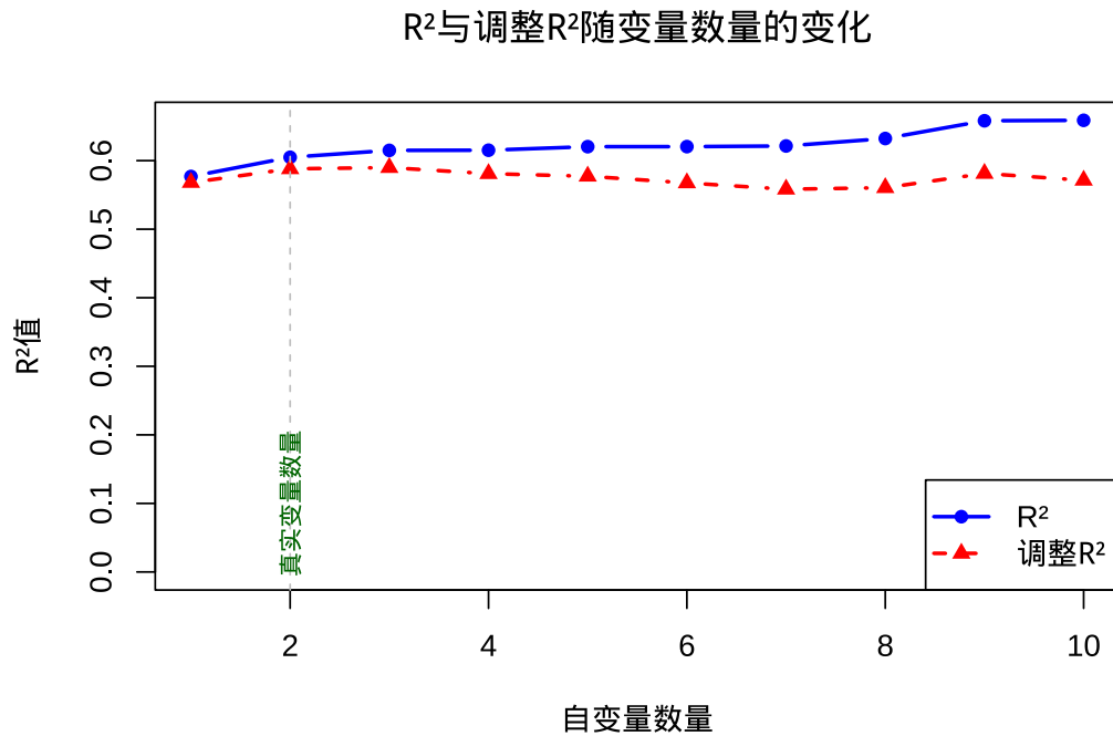
图 7.3 R^2 与调整 R^2 随自变量数量变化的对比：调整 R^2 对无关变量施加惩罚，防止过度拟合。
