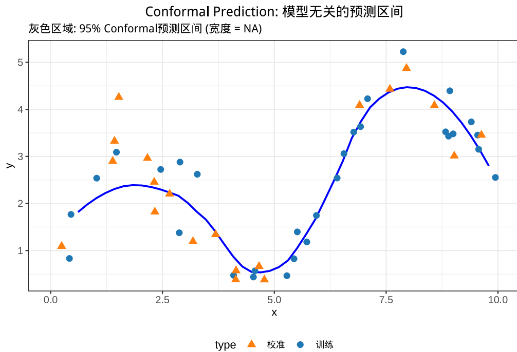
图 5.15 Conformal Prediction 预测区间演示：训练数据、校准数据、模型预测线和 95% 预测区间。区间宽度仅依赖于校准残差的分位数，与模型形式无关。
