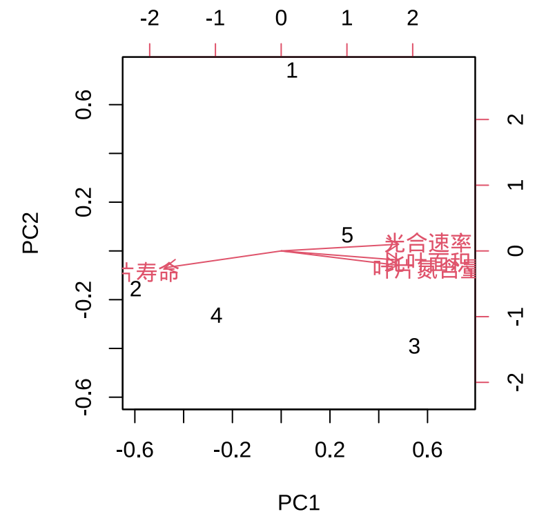
图 4.9 功能性状主成分分析的双标图：箭头表示各功能性状在前两个主成分上的载荷方向和大小，点表示物种在排序空间中的位置，物种间距离反映了功能性状的相似程度
