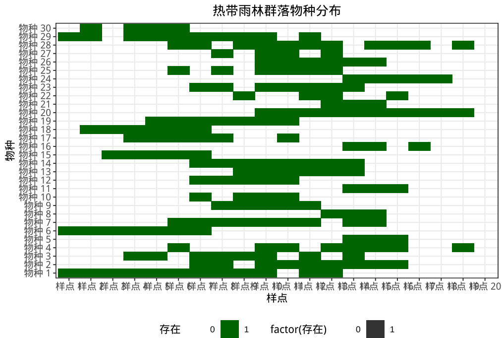
图 6.2 热带雨林群落物种分布热图：基于环境梯度的物种分布模式。使用颜色和透明度组合表示物种存在状态
