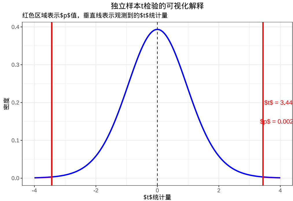
图 5.8 独立样本 t 检验的可视化解释：零假设下 t 分布、观测 t 统计量及 p 值区域。
