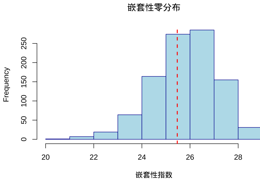
图 6.7 网络嵌套性零模型检验: 嵌套性指数零分布。使用虚线标识观测值位置, 确保在彩色显示和黑白打印时都能清晰识别
