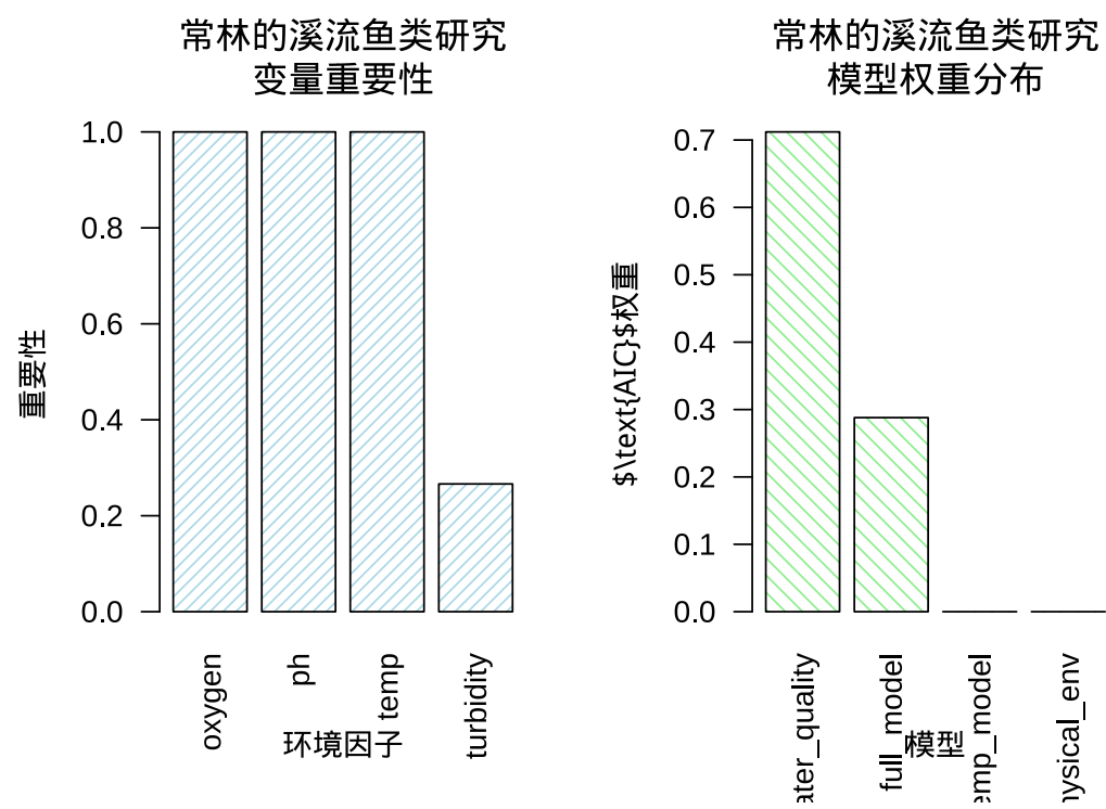
图 8.4 常林的溪流鱼类模型平均结果：变量重要性和模型权重分布。左图显示水温、溶解氧和 pH 值是影响鱼类丰度的关键因子，右图展示不同候选模型的相对支持度
