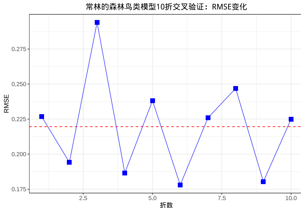
图 8.5 常林的森林鸟类模型 10 折交叉验证：RMSE 在不同数据子集上的变化。图中显示 RMSE 在不同折之间相对稳定，表明模型具有良好的泛化能力
