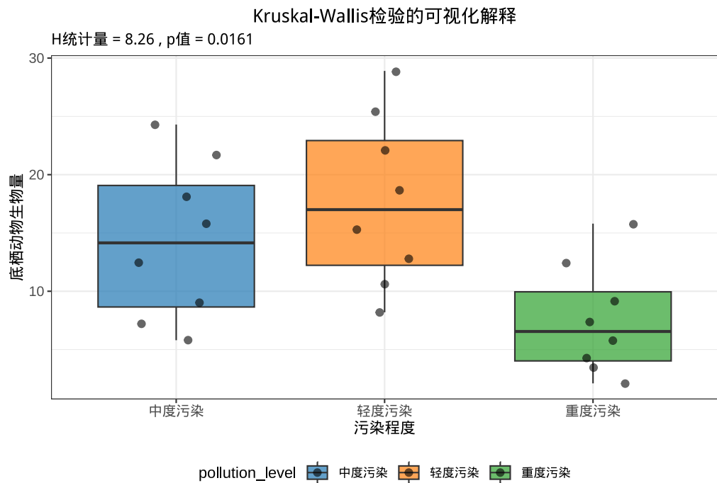
图 5.13 Kruskal-Wallis 检验的可视化解释：通过箱线图展示不同污染程度区域底栖动物生物量的分布比较 图5.13直观展示了 Kruskal-Wallis 检验的原理。箱线图显示了三个样本的分布情况，点表示各个观测值。检验基于这些观测值的秩次（排序位置）而不是原始数值来进行统计推断。
