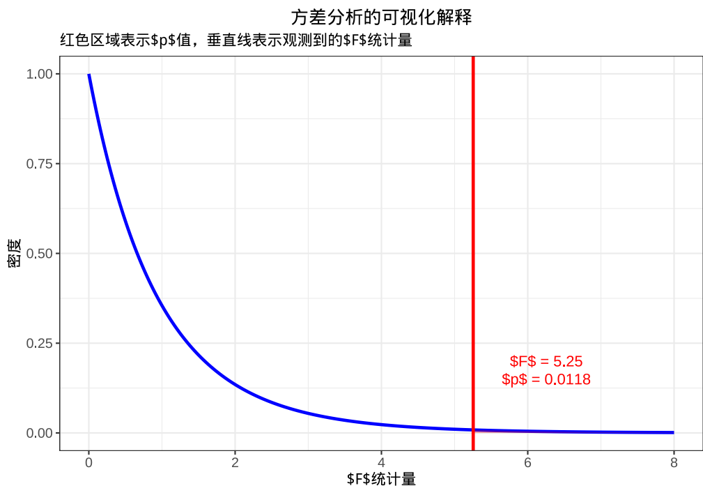
图 5.12 方差分析的可视化解：展示 F 分布、观测 F 统计量以及对应的 p 值区域
