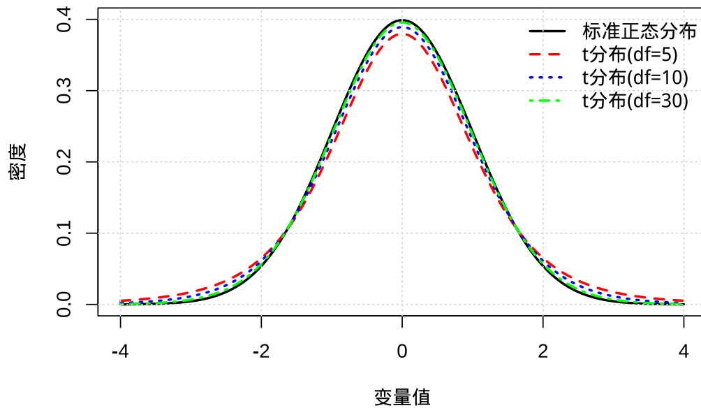
图 3.1 t 分布与正态分布的比较：随自由度增加，t 分布趋近标准正态分布。
