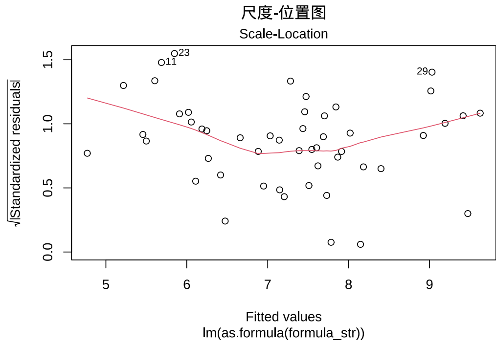
图 7.5 尺度-位置图：用于检查同方差性假设。
