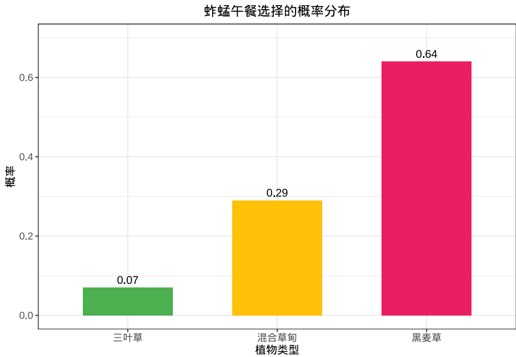
图 2.7 蚱蜢午餐选择的概率分布：三种草地的选择概率对比。
