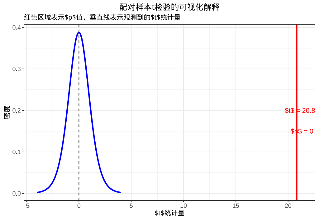
图 5.9 配对样本 t 检验的可视化解：配对差异均值的 t 分布、观测 t 统计量及 p 值区域。
