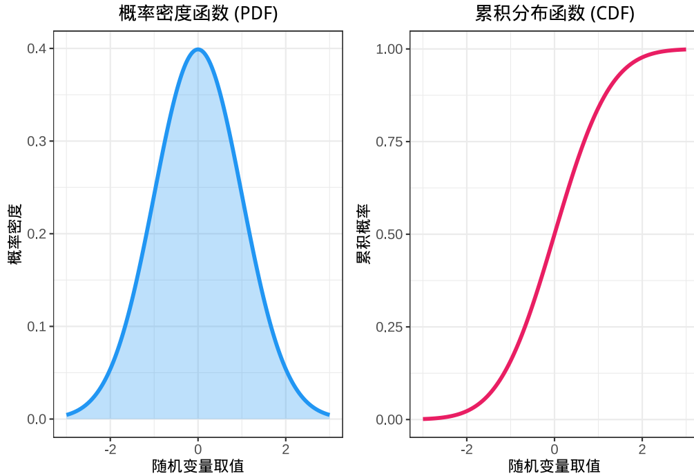
图 2.13 连续随机变量的概率密度函数与累积分布函数对比
