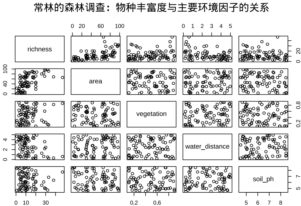
图 7.7 物种丰富度与主要环境因子的散点图矩阵，展示各变量间的两两关系，用于初步探索相关性和分布特征。
