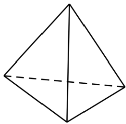
正四面体
