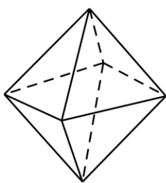
正八面体
