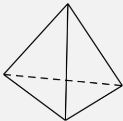
正四面体
