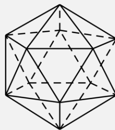
正二十面体
