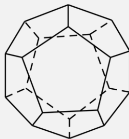
正十二面体
