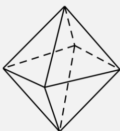
正八面体
