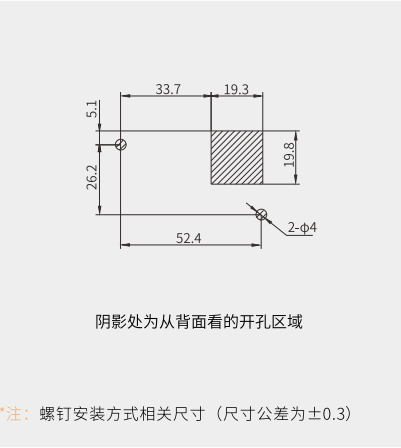
① 建议螺丝安装尺寸
