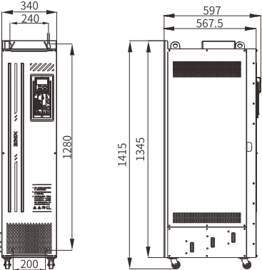
X9机型: 315~450kW
