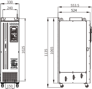
X7机型: 185~220kW
