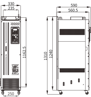
X8机型: 250~280kW
