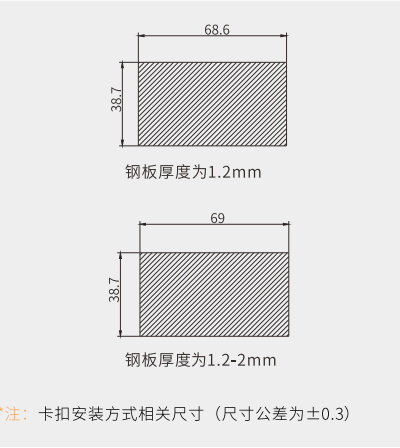
② 建议卡扣安装尺寸
