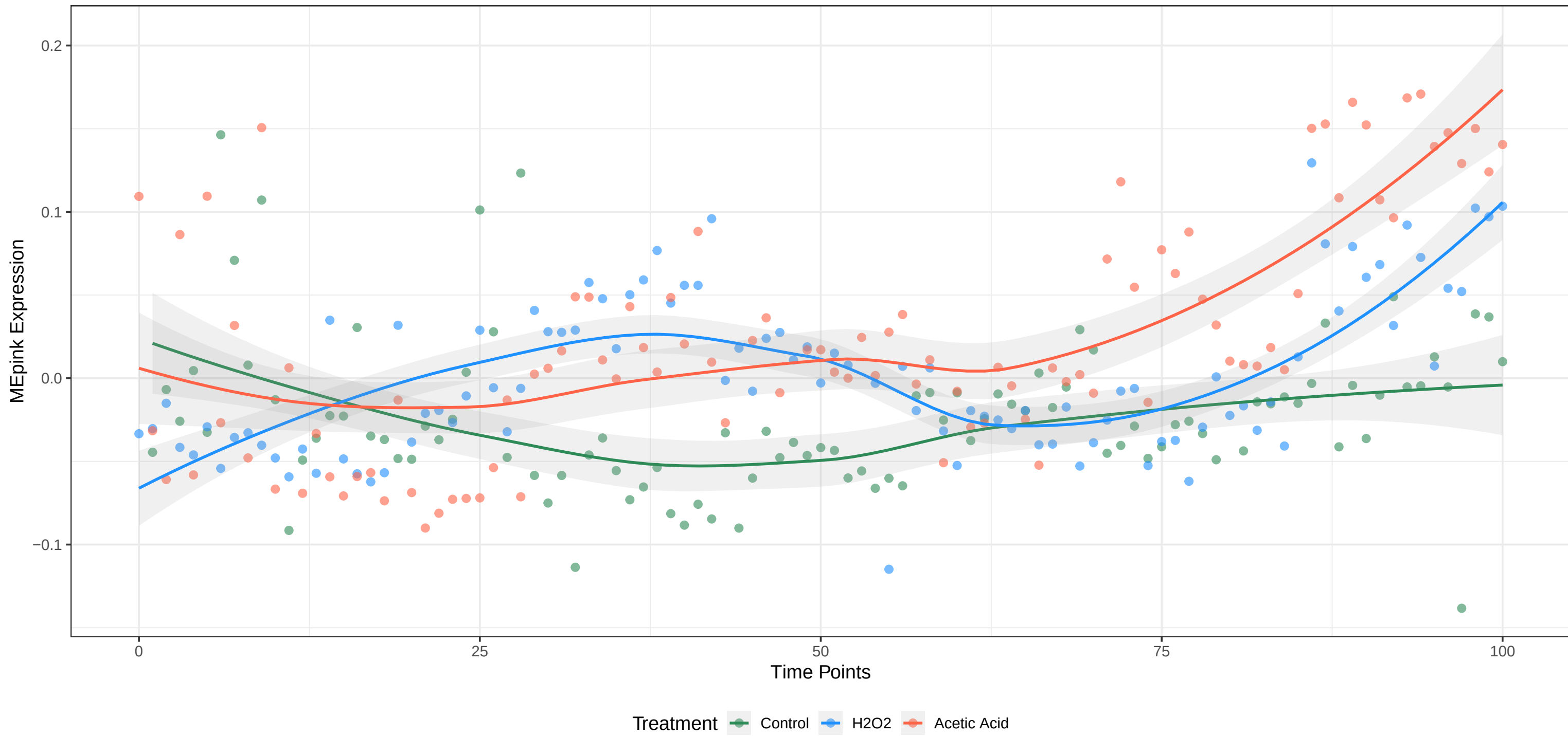
MEpink Module Eigengene Dynamics
