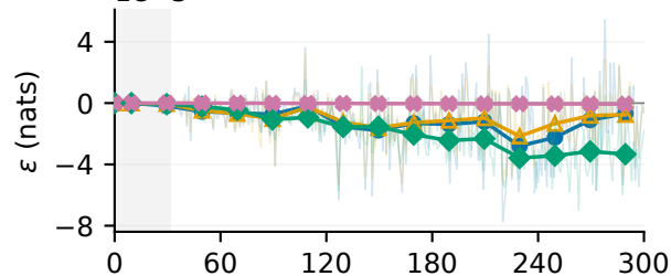
1e-3 (d) Remaining response \varepsilon
