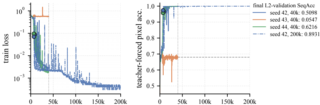
(d) d256, 8 layers, 4 heads, 6,581,505 parameters
