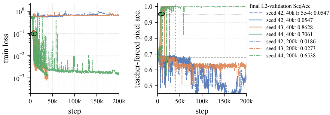
(d) d256, 8 layers, 4 heads, 6,581,505 parameters
