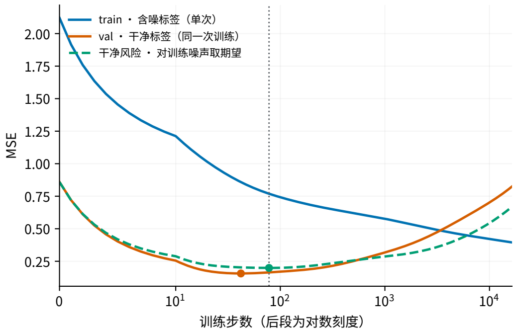
n=64, \sigma^2=1 , seed 414 实际 val 最低点 42 步；期望风险最低点 78 步
