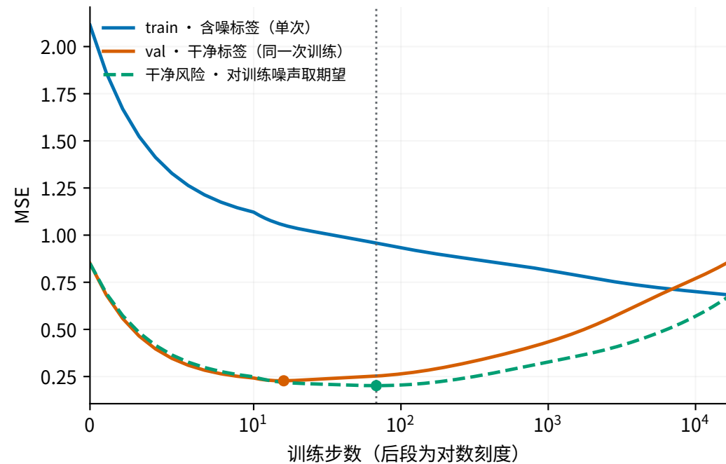
n=64, \sigma^2=1 , seed 411 实际 val 最低点 16 步；期望风险最低点 68 步
