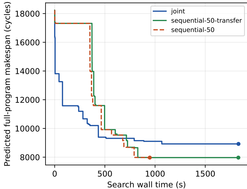
LU
