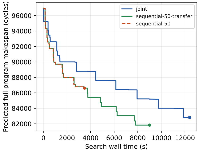
GCN
