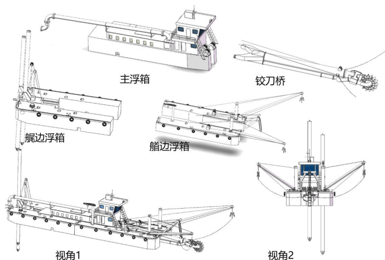
模块化环保绞吸船设计
