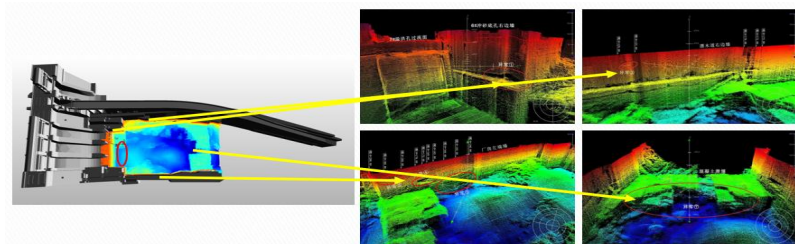
三维数字化点云
