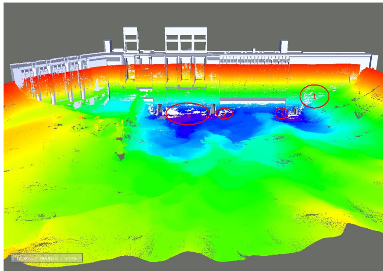
上游坝面混凝土表观完整情况检测
