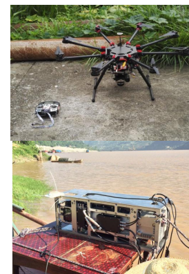
无人机、车、船搭载进行扫描
