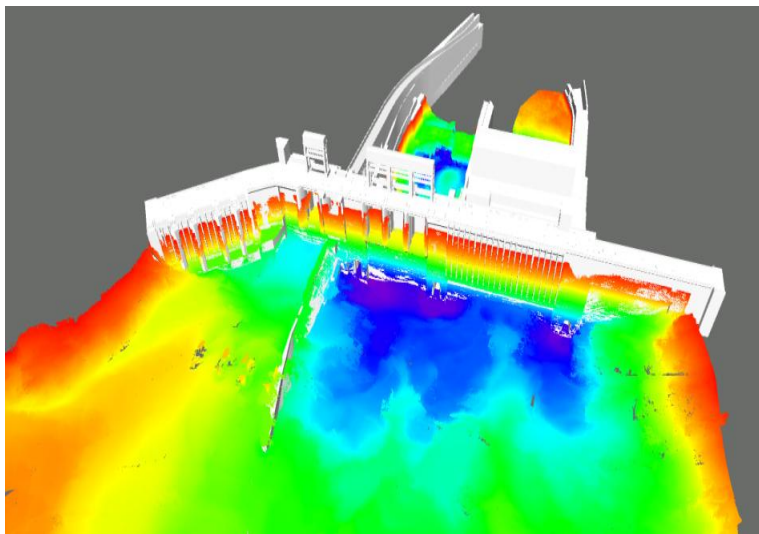
尾水渠水下检测成果
