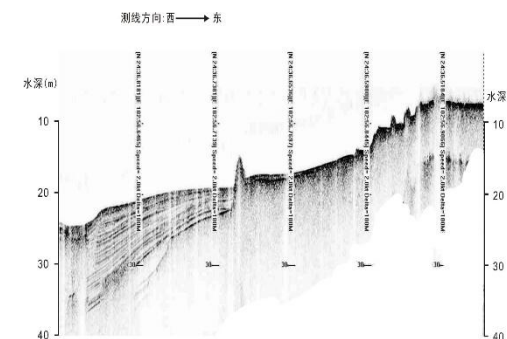
浅地层剖面探测技术
