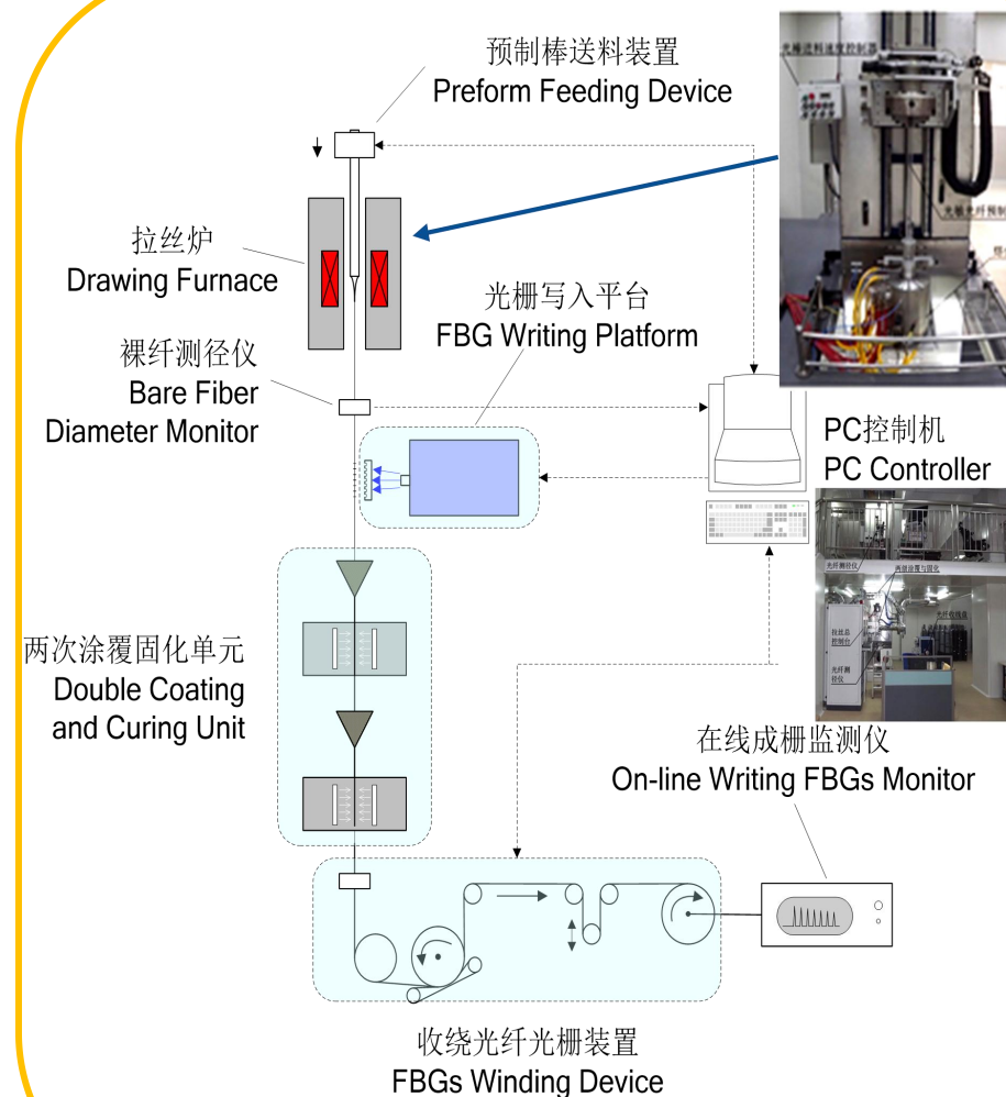
光栅阵列制备技术
