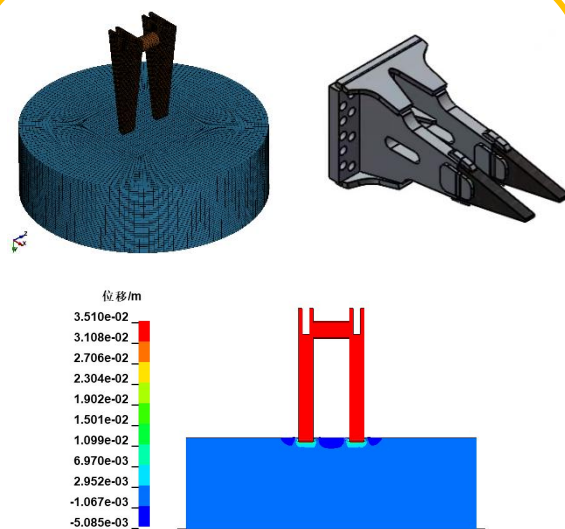
高频碎岩锤数值模拟
