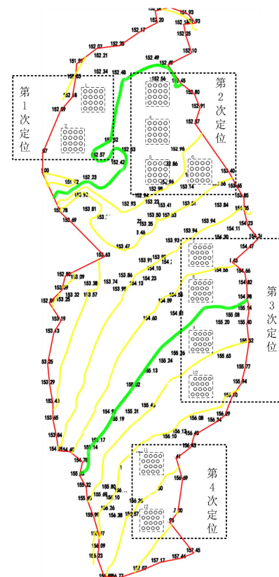
布点方案与三维重构法绘制水下地形
