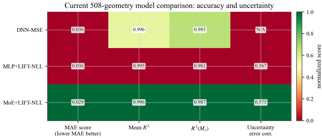
图 2-8 当前 508 几何上的模型精度与不确定度对比热力图。MAE score 表示对 MAE 反向归一化后的得分，数值越高表示点误差越低；uncertainty error corr. 为样本平均绝对误差与预测不确定度之间的相关性，DNN 无不确定度输出，记为 N/A。
