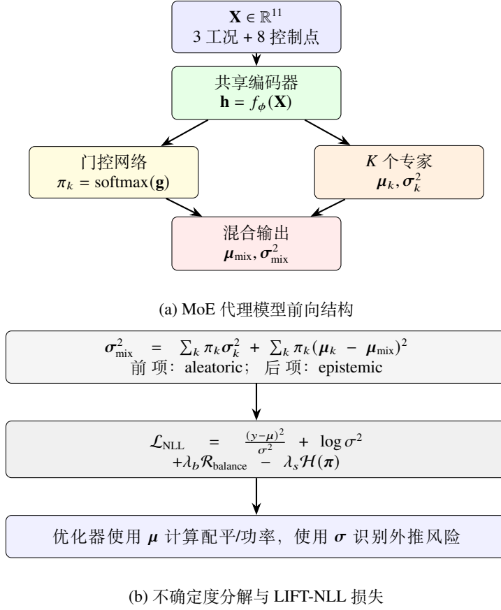
图 2-6 MoE + LIFT-NLL 网络架构与损失机制。为避免单幅图中过多连线重叠，图中将模型前向结构和不确定度/损失机制分为两个子图表示。
