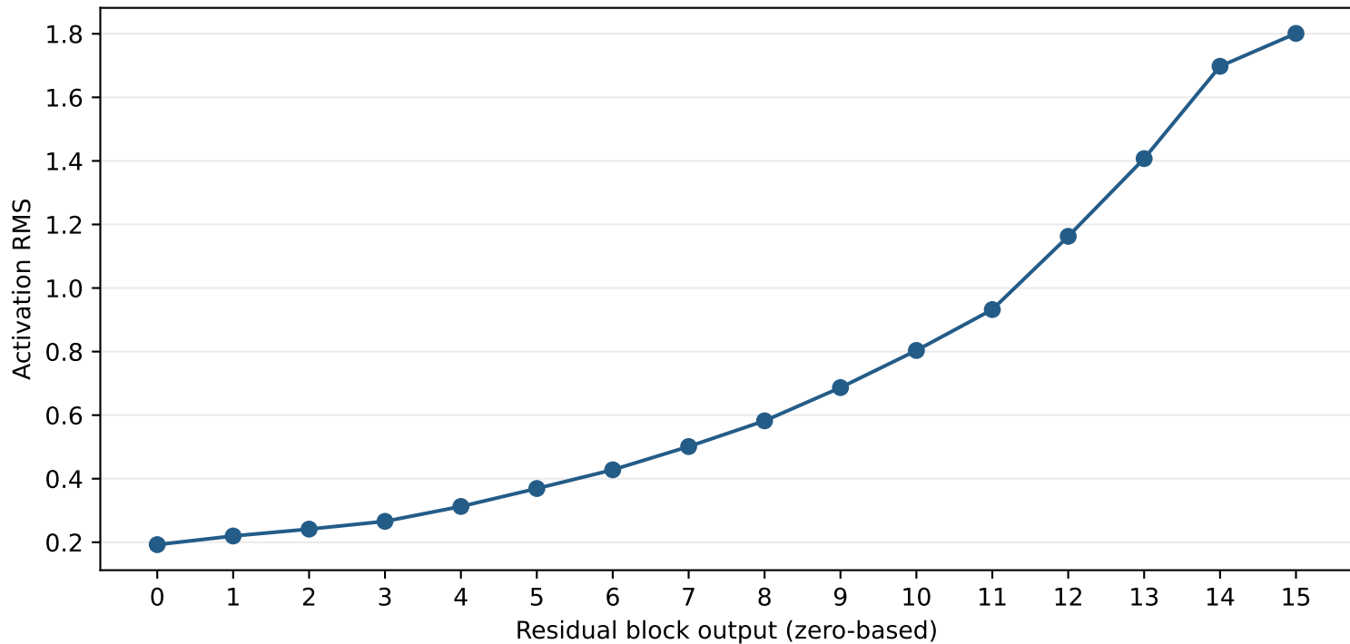
MIRA Mini 4P: all-layer capture sanity check
