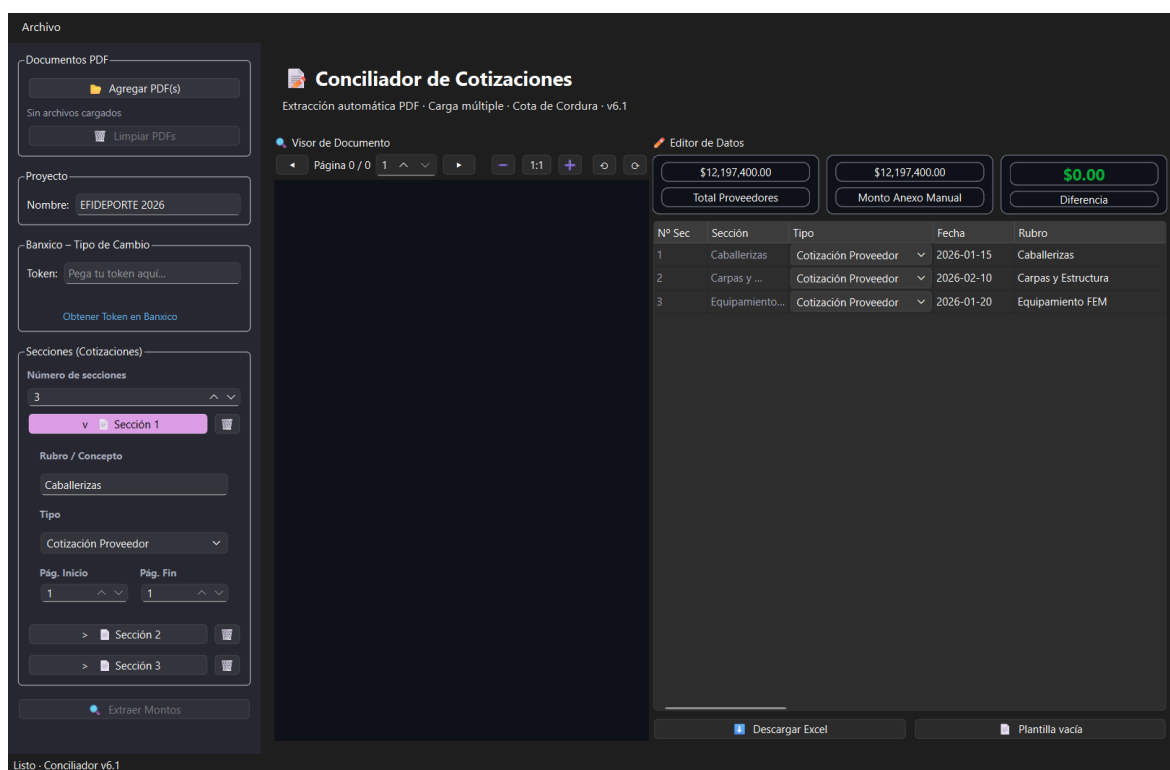
Figura 4.2: Vista completa después de la extracción: visor PDF + tabla con resultados.
