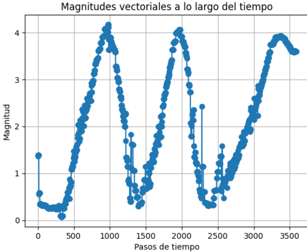
Figura 1: Gráfica de la magnitud del vector de posición a lo largo del tiempo, mostrando el jitter observado durante la trilateración 2D.
