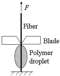
Micro-bond test
