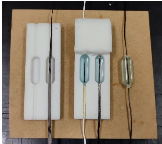
Figura 3.3 Secuencia de fabricación de probetas FBPO: cavidad de silicona, posicionamiento de hebra, colado/curado y desmoldeo.
