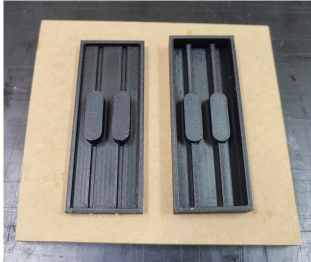
Figura 3.1 Molde negativo impreso en PLA (multicavidad) con canales y topes geométricos para fijar \ell_e .
