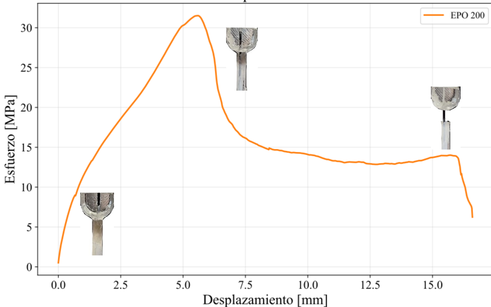
Esfuerzo vs Desplazamiento - EPO 200
