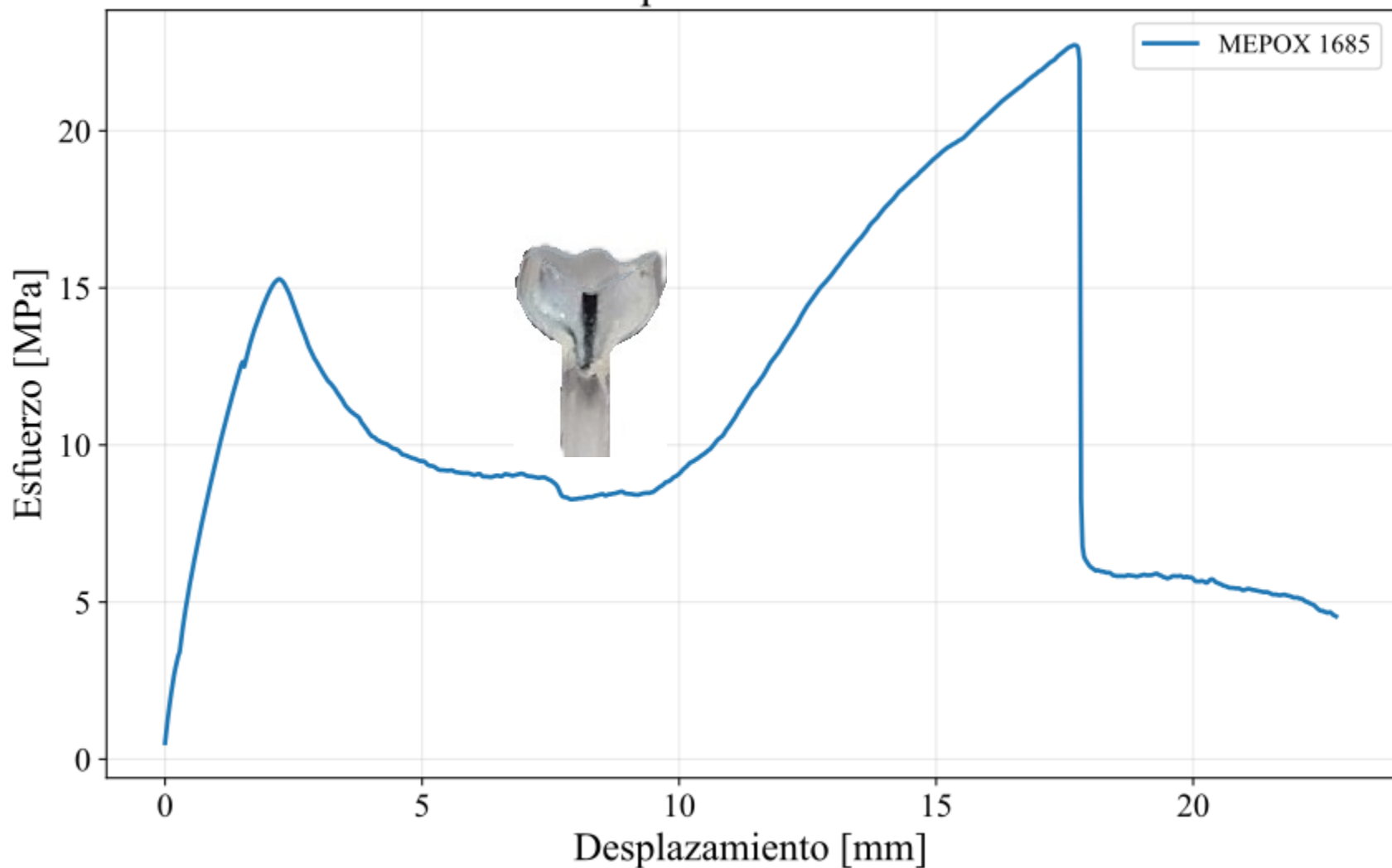
Esfuerzo vs Desplazamiento - MEPOX 1685
