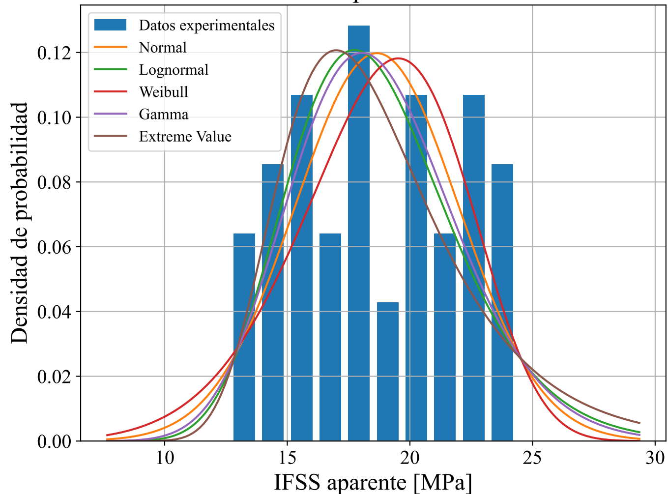
Distribución IFSS aparente MEPOX - HTA
