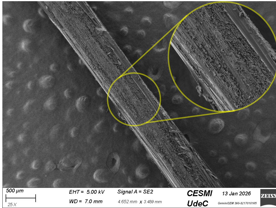
Figura 2.3 Micrografía SEM representativa de la interfaz fibra - matriz, donde se observa la superficie de una hebra de fibra tras un ensayo de tipo Fiber-Bundle Pull-Out .
