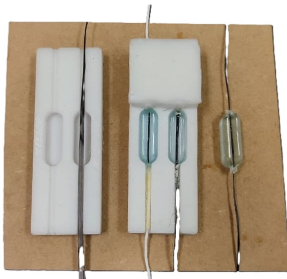
Figura 3.5 Secuencia de fabricación de probetas FBPO: (a) cavidad de silicona, (b) posicionamiento de la hebra, (c) colado y curado de la resina y (d) probeta desmoldeada.
