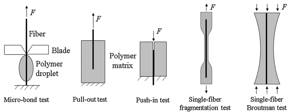
Figura 2.5 Tipos de ensayo para la caracterización interfacial.
