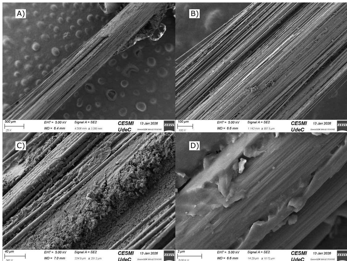
Figura 4.6 micrografías SEM de A) Probeta EPO-HTA, B) Acercamiento zona de la interfase, C) Acercamiento a varios filamentos, D) Acercamiento a filamento individuales.
