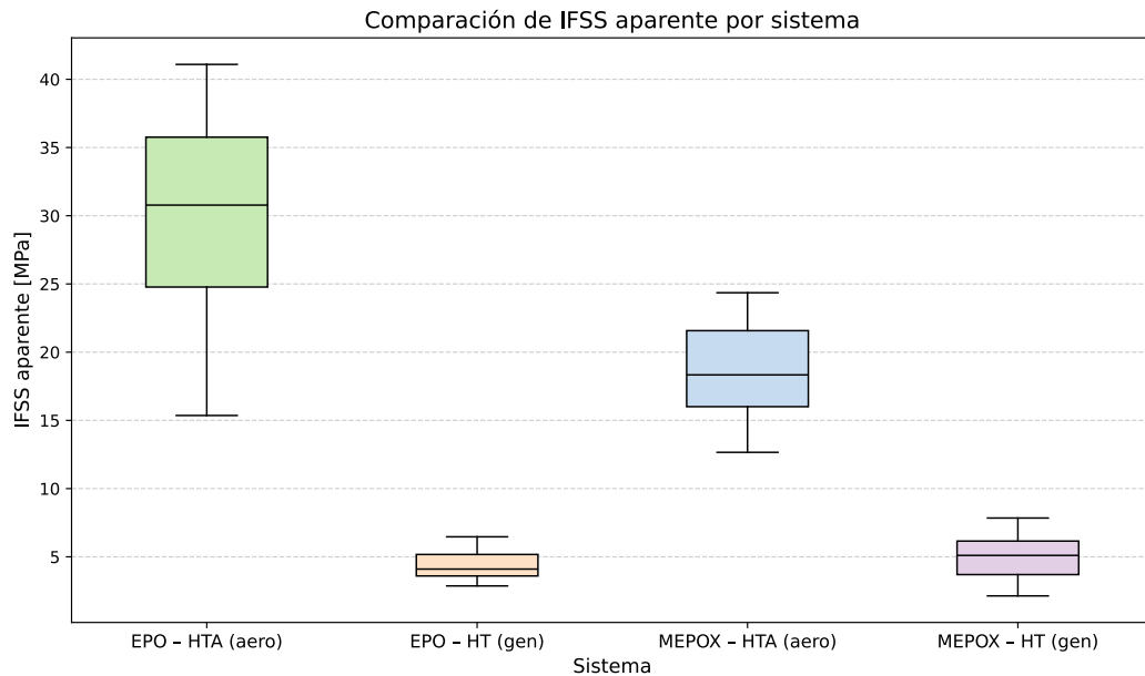
Figura 4.10 Boxplot de los valores de IFSS aparente obtenidos para los sistemas evaluados.
