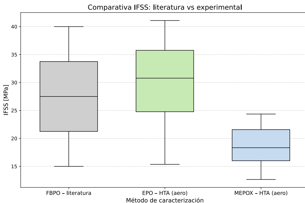
Figura 4.11 Comparación entre los valores de IFSS aparente obtenidos experimentalmente en este estudio y los rangos de IFSS reportados en la literatura para ensayos FBPO.
