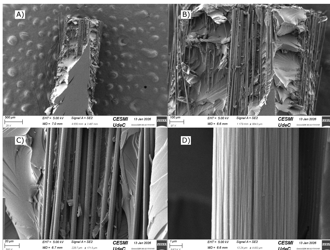
Figura 4.5 micrografías SEM de A) Probeta MEPOX-HTA, B) Acercamiento zona de la interfase, C) Acercamiento a varios filamentos, D) Acercamiento a filamento individuales.
