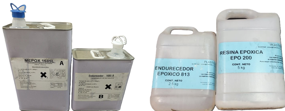
Figura 3.6 Sistemas epoxi de baja viscosidad utilizados en este estudio. Izquierda: MEPOX 1685L. Derecha: EPO 200.
