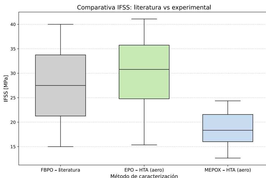
Figura 4.7 Comparación entre los valores de IFSS aparente obtenidos experimentalmente en este estudio y los rangos de IFSS reportados en la literatura para ensayos FBPO.
