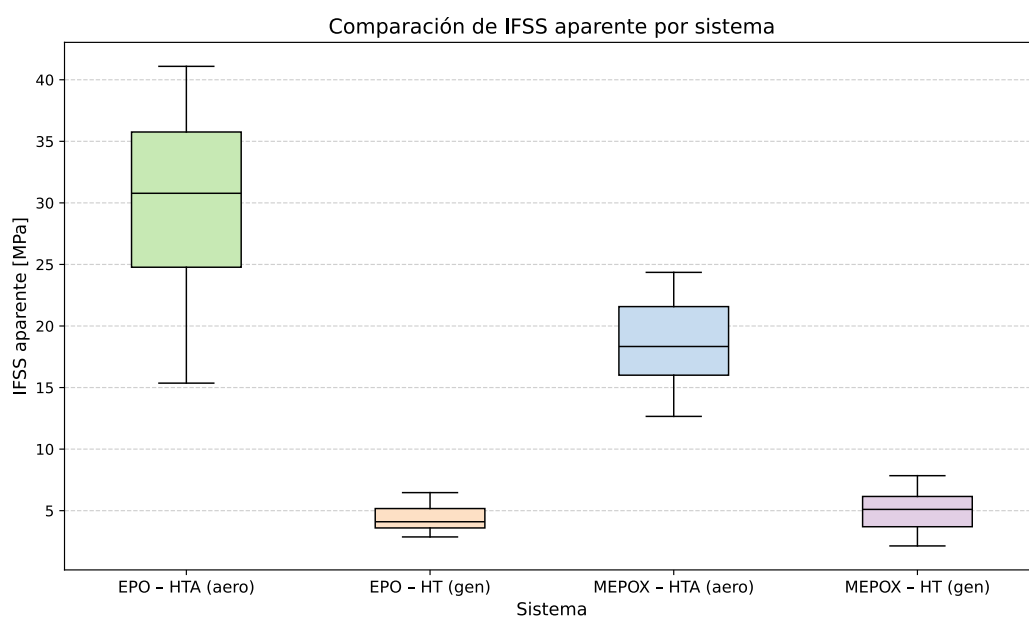
Figura 4.6 Boxplot de los valores de IFSS aparente obtenidos para los sistemas evaluados.
