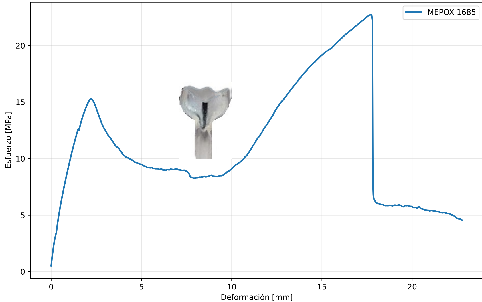
Esfuerzo vs Deformación - Ensayo FBPO
