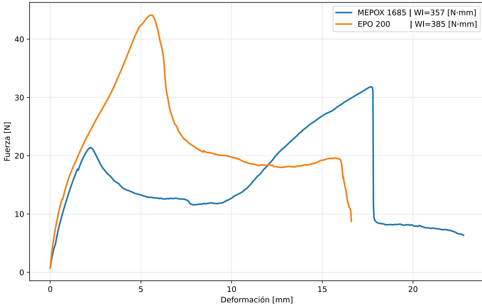
Fuerza vs Deformación - Ensayo FBPO
