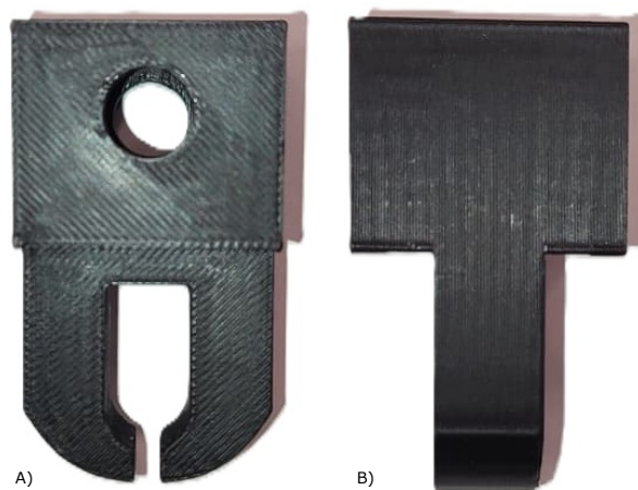
Figura 3.8 Mordaza diseñada para el ensayo FBPO: (A) vista frontal, mostrando la geometría de sujeción de la hebra; (B) vista lateral.
