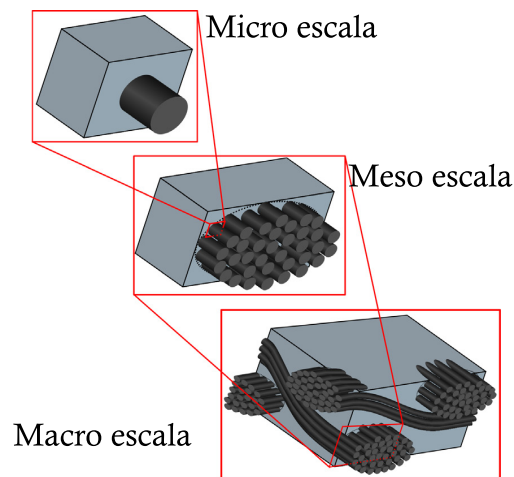
Figura 2.3 Escalas de estudio en materiales compuestos reforzados con fibra.
