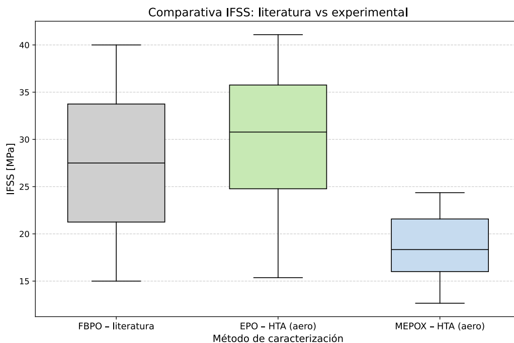
Figura 4.9 Comparación entre los valores de IFSS aparente obtenidos experimentalmente en este estudio y los rangos de IFSS reportados en la literatura para ensayos FBPO.
