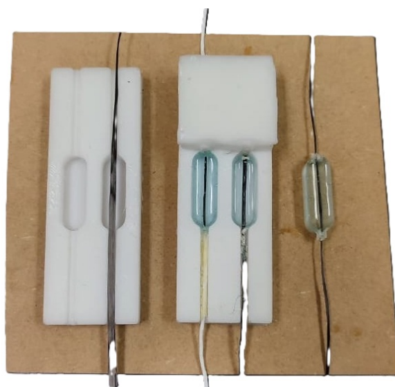
Figura 3.5 Secuencia de fabricación de probetas FBPO: (a) cavidad de silicona, (b) posicionamiento de la hebra, (c) colado y curado de la resina y (d) probeta desmoldeada.
