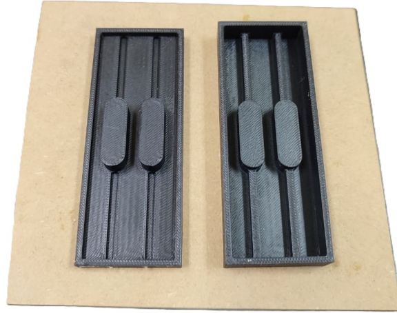
Figura 3.3 Molde negativo impreso en PLA (arquitectura multicavidad) con canales de sección constante y topes geométricos integrados para fijar la longitud de embebido \ell_e .
