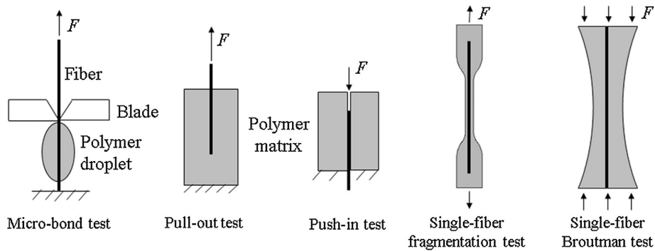
Figura 2.4 Tipos de ensayo para la caracterización interfacial.
