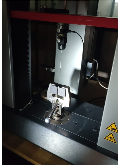
Figura 3.7 Montaje experimental del ensayo Fiber-Bundle Pull-Out (FBPO).
