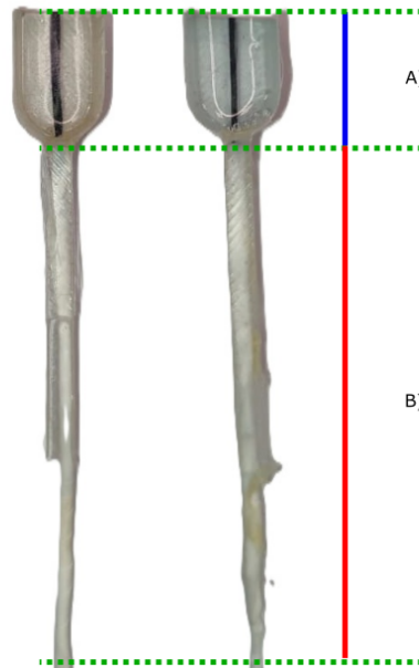
Figura 4.1 Identificación de regiones en una probeta FBPO: (A) región embebida asociada al despegue interfacial y (B) región de hebra libre dominada por fricción y sujeción.
