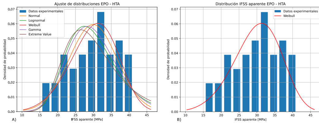
Figura 4.10 Comparación de distribución para IFSS aparente del sistema EPO-HTA. A) Ajuste para diferentes curvas teóricas. B) Ajuste utilizando Weibull.
