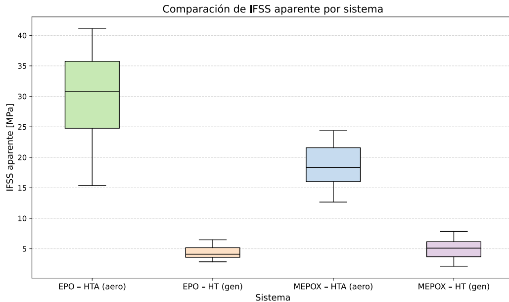
Figura 4.8 Boxplot de los valores de IFSS aparente obtenidos para los sistemas evaluados.
