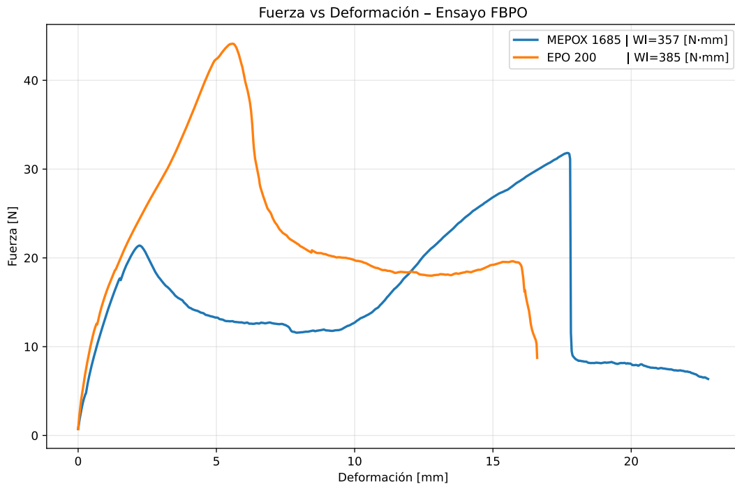
Figura 4.5 Curvas fuerza - desplazamiento representativas obtenidas durante los ensayos FBPO para los sistemas fibra - matriz evaluados.
