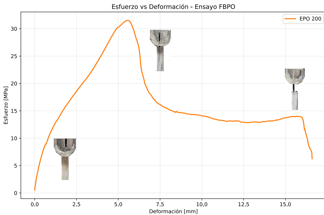
Figura 4.6 Curvas esfuerzo - desplazamiento con registro de las etapas del ensayo.
