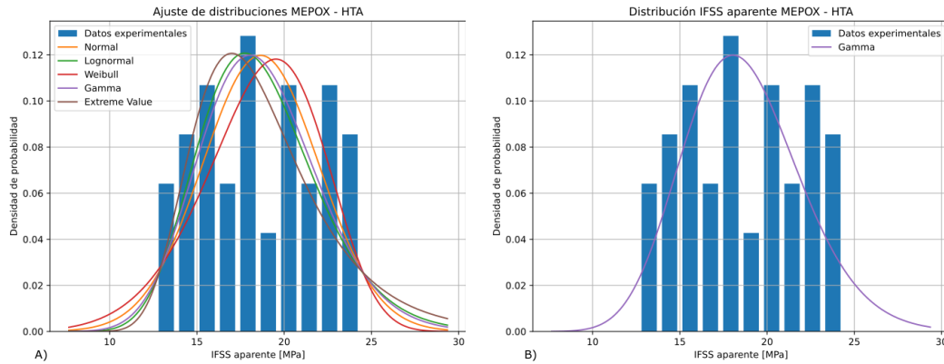
Figura 4.11 Comparación de distribución para IFSS aparente del sistema MEPOX-HTA. A) Ajuste para diferentes curvas teóricas. B) Ajuste utilizando Gamma.
