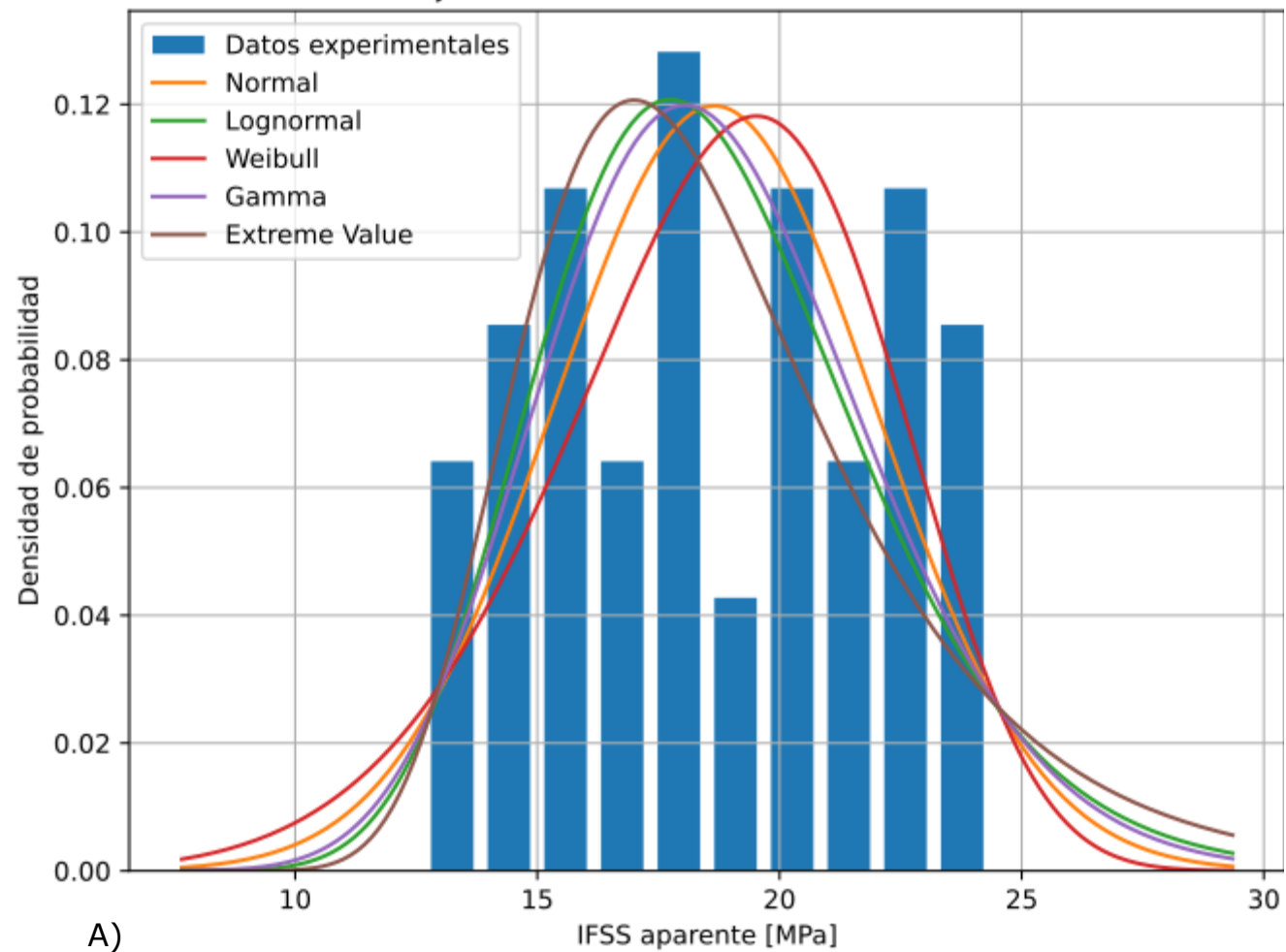
Ajuste de distribuciones MEPOX - HTA
