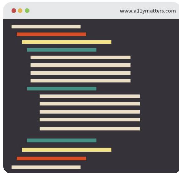
DOM
